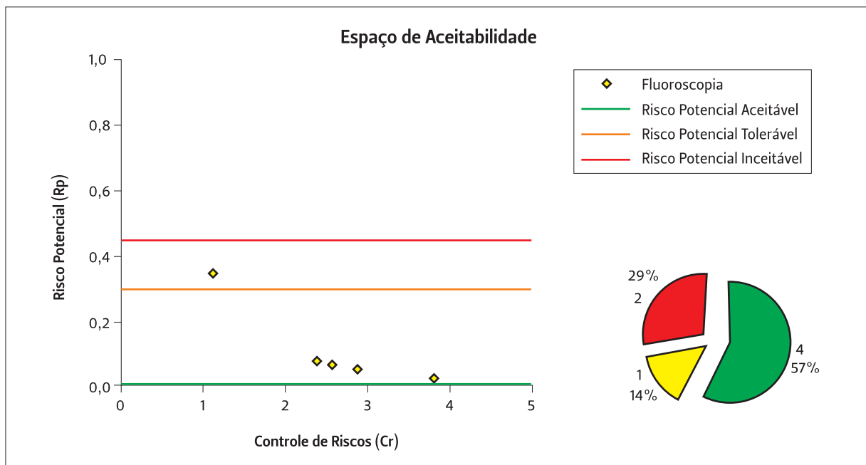
FIGURA 5 – GRÁFICO DO ESPAÇO DE ACEITABILIDADE EM PROCEDIMENTO DE FLUOROSCOPIA
