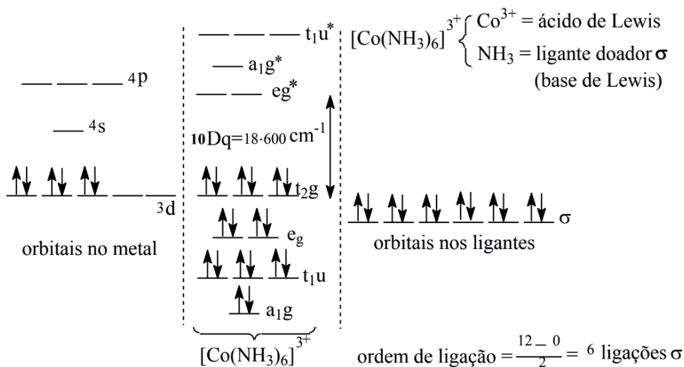
Figura 29 – Diagrama qualitativo de orbital molecular para o complexo [\text{Co}(\text{NH}_3)_6]^{3+}
