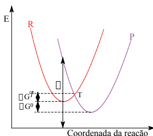
Figura 74 – Representação do perfil de uma reação de transferência de elétrons de esfera externa com destaque para os parâmetros \lambda , \Delta G^* e \Delta G^0 . T (ou ^\ddagger ) representa o estado de transição para a reação
