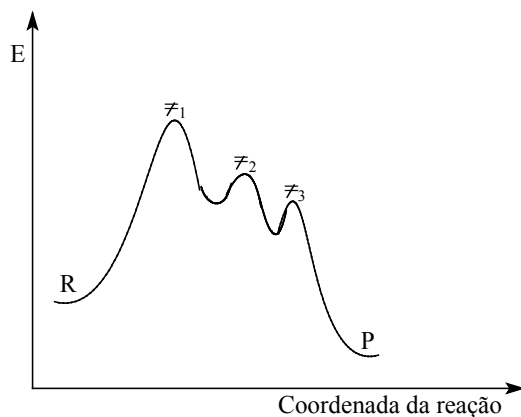
Figura 69 - Representação do perfil de uma reação de transferência de elétrons via esfera interna em que a formação do complexo precursor é a etapa lenta ( \neq_1 ) no processo (a)
