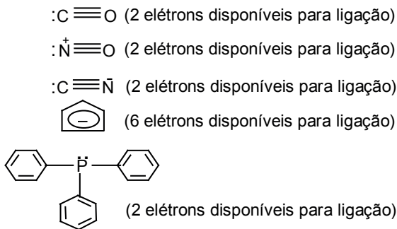
Figura 7 – Representação da estrutura dos ligantes CO, NO + , CN - , C 5 H 5 - e PØ 3
