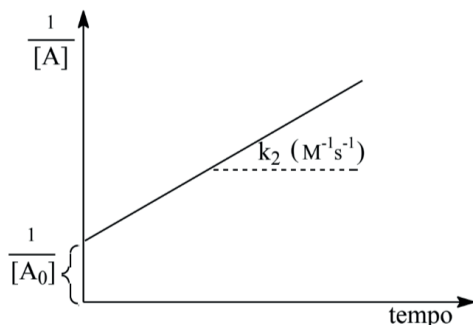
Figura 47 - Representação do gráfico de 1/[A] versus o tempo para uma reação de segunda ordem, em que K_2 = constante de velocidade para a reação
