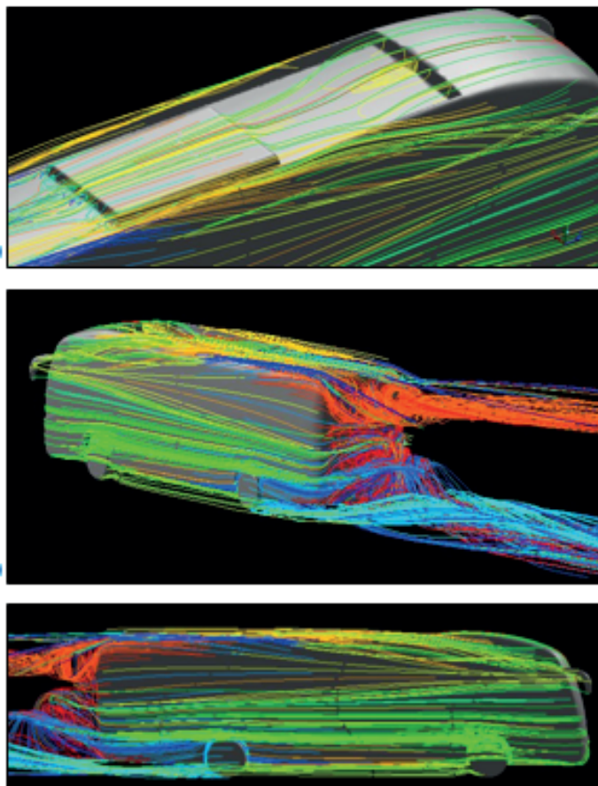
Figura 18 – Linhas de corrente para o modelo do ônibus em escala 1/24.
