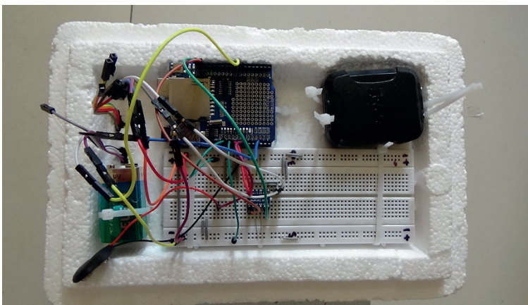
Figura 3 – Parte interna da tampa do Payload, montado com sensores e placa de Arduino.
