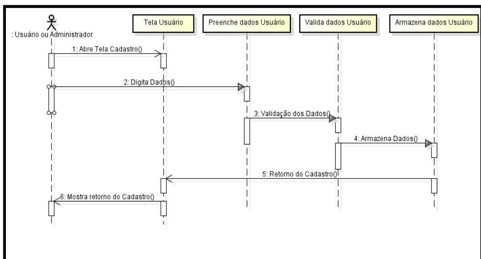
Figura 19 – Diagrama de sequência cadastrar usuário WebApp Turminha UNA (Autores, 2023).
