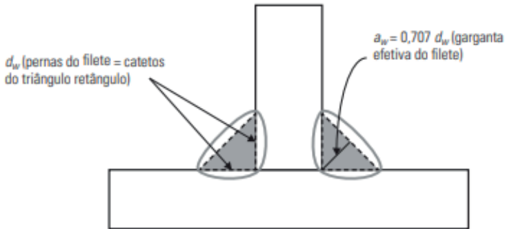
Figura 37: Representação Solda de Filete
