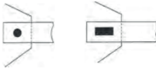
Figura 39: Representação solda de tampão
