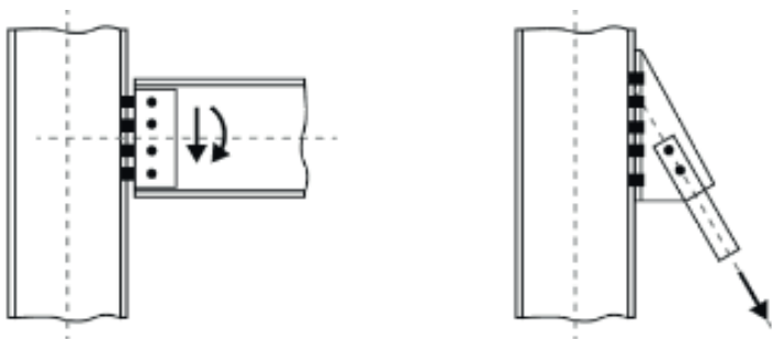
Figura 31: Esforços combinados tração + cisalhamento
