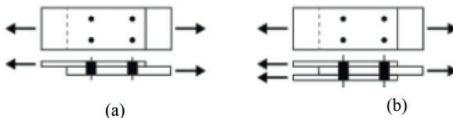
Figura 29 (a) Cisalhamento centrado simples (b) Cisalhamento centrado duplo
