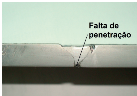
Figura 46: Cordão de solda com falta de penetração
