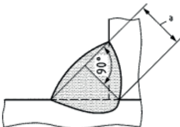
Figura 52: Espessura da garganta com penetração
