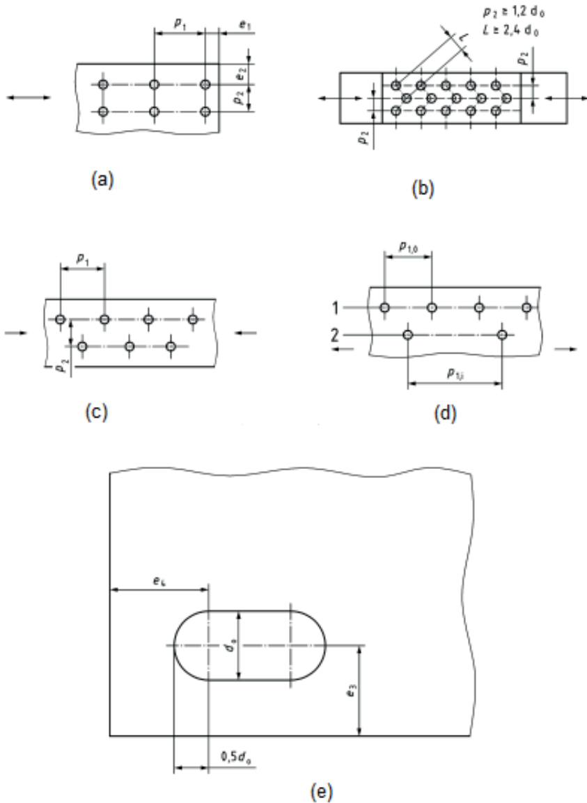
Figura 49: Símbolos para distância a borda e espaçamento de fixadores
