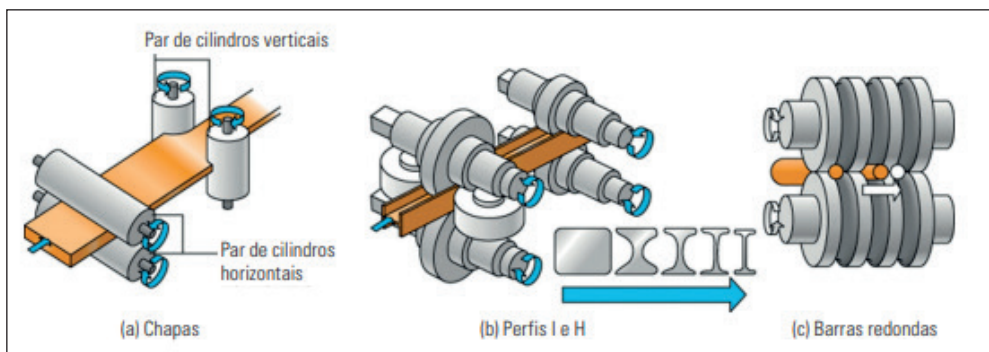
Figura 1: (a) Laminação chapas; (b) Laminação Perfis; (c) Laminação barras redondas
