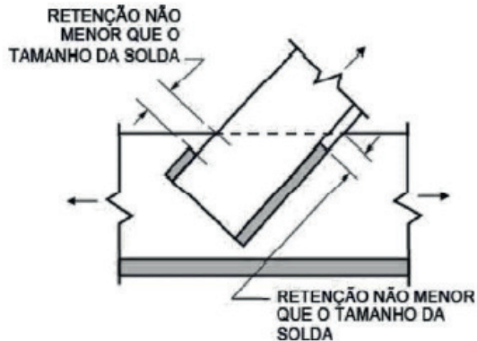
Figura 53: Terminação de soldas de sobreposição
