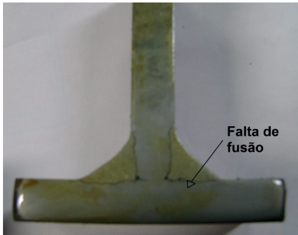
Figura 45: Cordão de solda com falta de fusão
