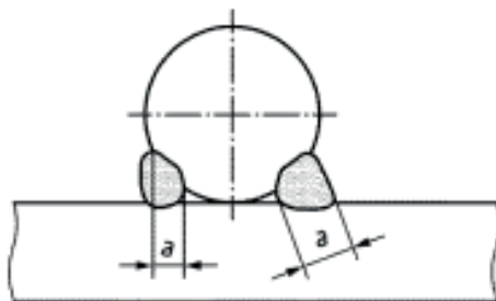
Figura 50: Espessura da garganta de soldas de chanfro em seções sólidas
