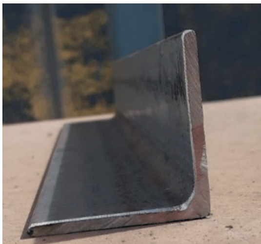
Figura 3: Cantoneiras de abas iguais
