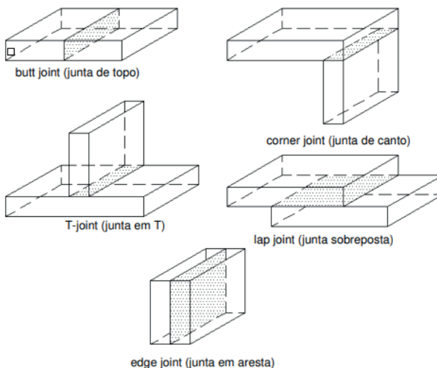
Figura 40: Tipos de Juntas
