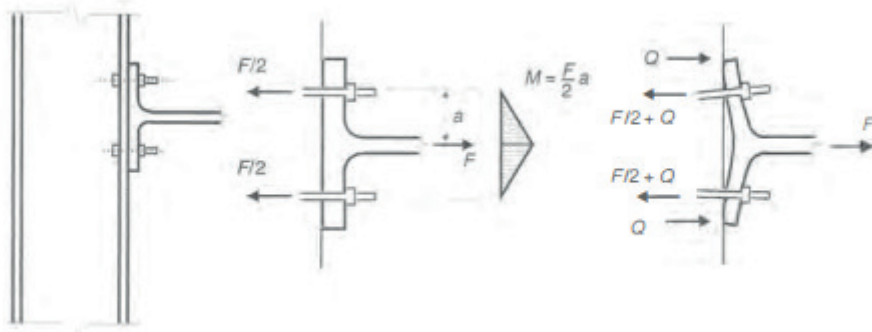
Figura 28: Ligação com parafusos sujeitos à esforço de tração
