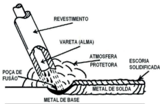
Figura 32: Arco elétrico com eletrodo revestido
