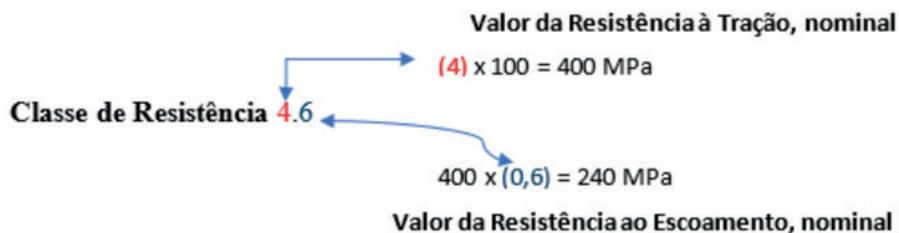
Figura 25: Significado dos números das classes dos parafusos da Norma ISO
