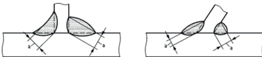
Figura 51: Espessura garganta efetiva solda de filete
