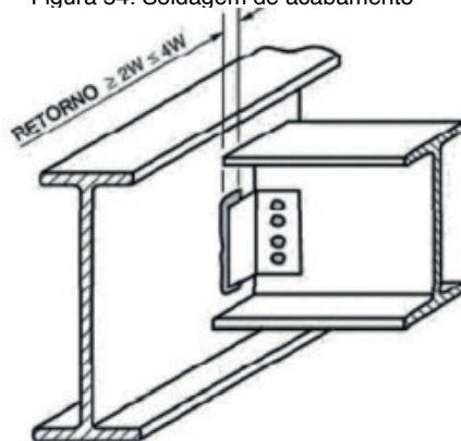
Figura 54: Soldagem de acabamento
