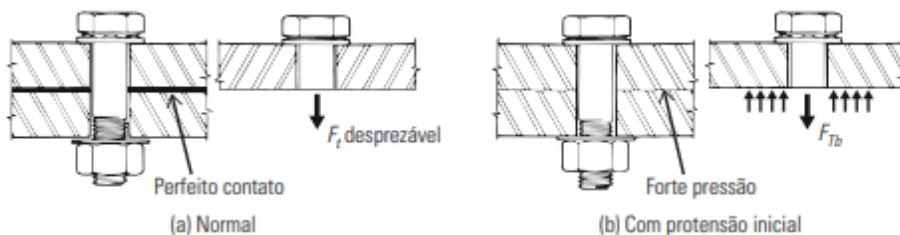
Figura 27: Tipos de aperto aplicados nos parafusos de alta resistência
