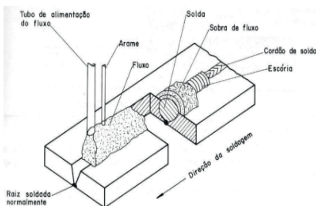
Figura 36: Soldagem ao Arco Submerso
