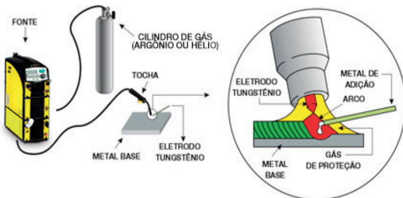
Figura 35: Soldagem com eletrodo de Tungstênio (TIG)
