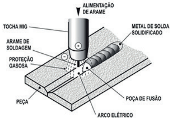
Figura 34: Soldagem a arco gás com tocha MIG
