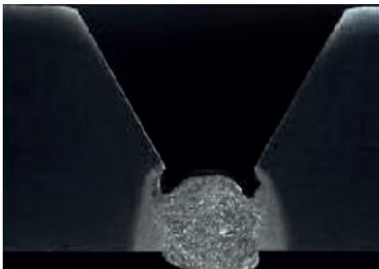
Figura 47: Presença de descontinuidade de mordeduras
