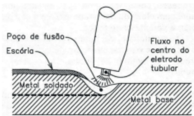
Figura 33: Soldagem arame tubular
