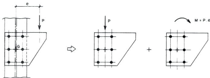
Figura 30: Parafuso sob cisalhamento excêntrico
