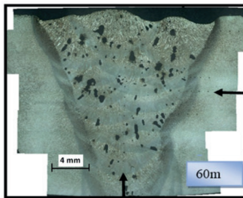
Figura 44:Cordão de solda com inclusão de escória
