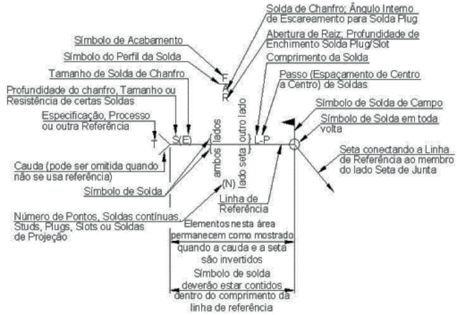
Figura 42: Símbolo soldagem
