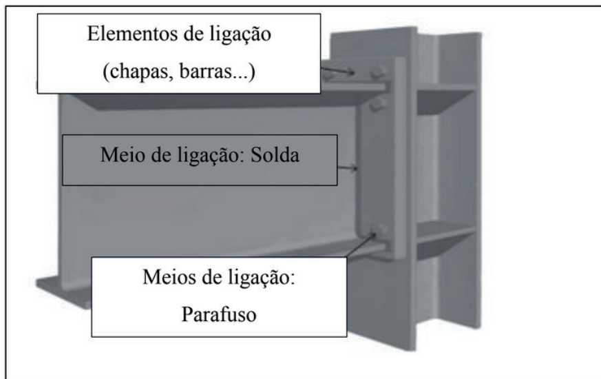
Figura 24: Elementos de ligação e Meios de ligação
