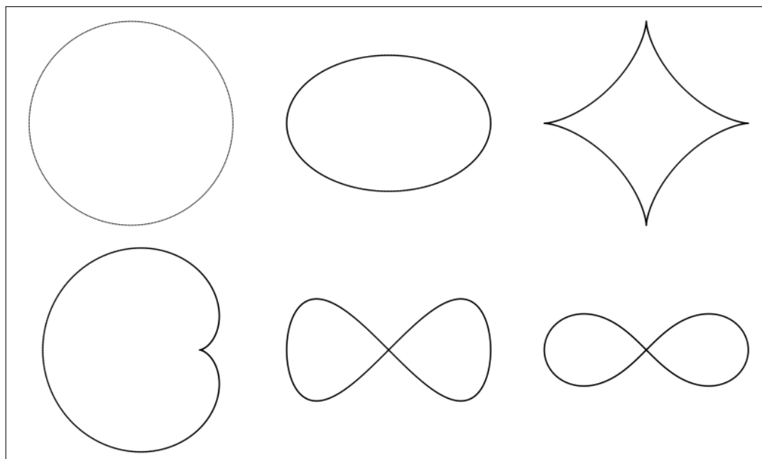
Figura 5.2: Curvas planas: circunferência, elipse, astroide, cardioide, lemniscata de Geronon e lemniscata de Bernoulli.
