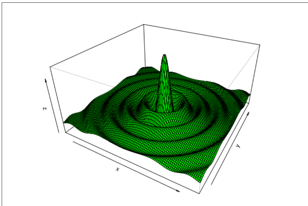
Figura 5.1: Gráfico da função f : \mathbb{R} \rightarrow \mathbb{R} \quad f(x, y) = \frac{\sin(\sqrt{x^2+y^2})}{\sqrt{x^2+y^2}} .
