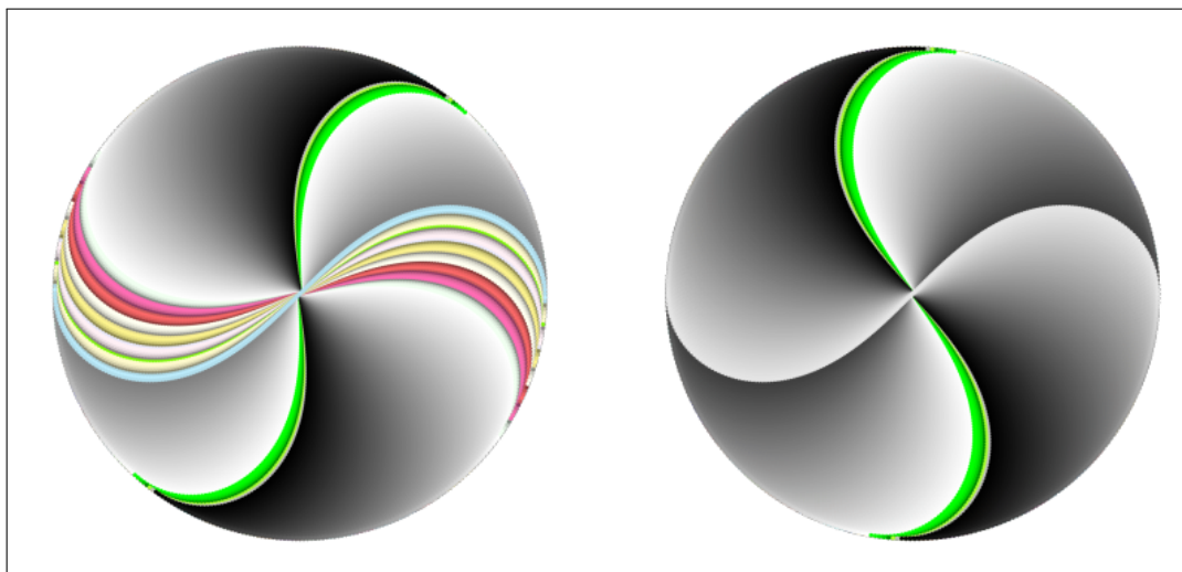
Figura 5.13: Rotações sucessivas da Lemniscata de Bernoulli para t \in [0, \pi] .
