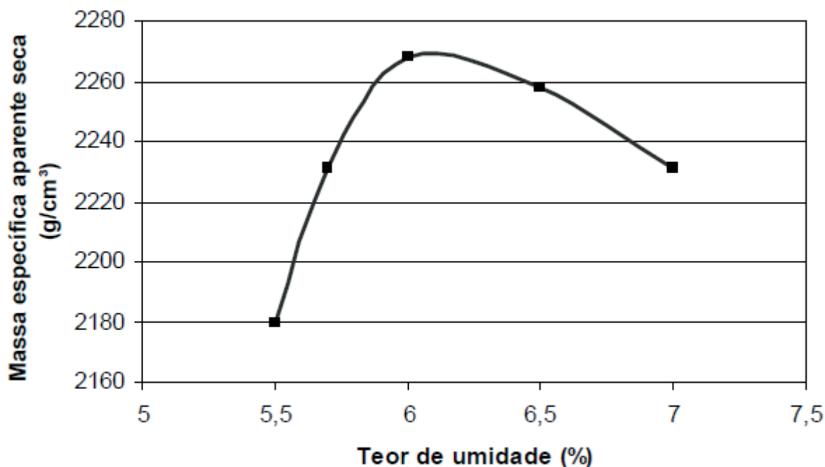
Figura 44 – Curva de compactação do CCR, consumo de cimento 110 kg/m³. Extraído de Ricci [79].
