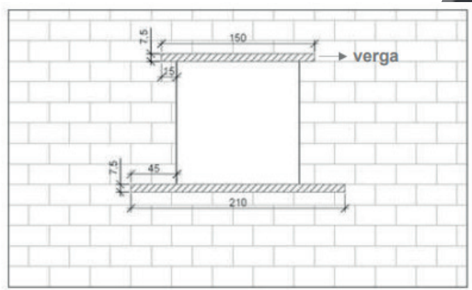
Figura 51 – Execução de vergas e contravergas em alvenarias. Fonte: google imagens.
