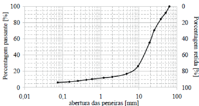
Figura 10 – O ensaio de peneiramento consiste em agrupar peneiras em ordem crescente, e medir a massas percentuais retidas, ou passantes, acumuladas, construindo um gráfico em função do tamanho de tela de aberturas das peneiras.
