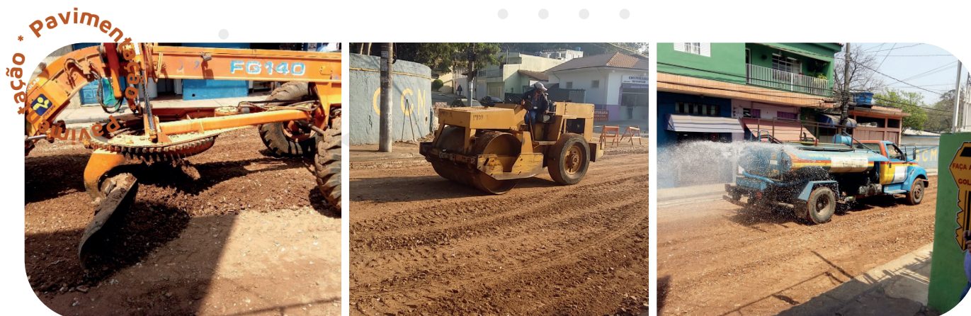
Figura 20 – Sequência de execução de uma sub-base de pavimento flexível com bica corrida reciclada mista. Fonte: IPT.
