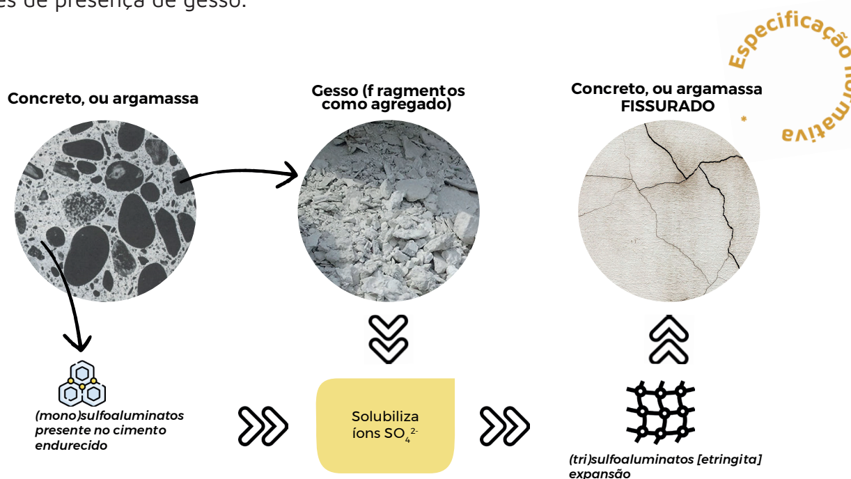
Figura 11 – Mecanismo de fissuração do concreto pela presença de fração de gesso no AR. Fonte: imagem à esquerda extraída de [15], as demais obtidas no banco do google imagens.
