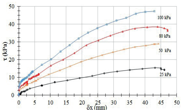
Figura 9: Deslocamento horizontal versus tensão cisalhante - M100%
