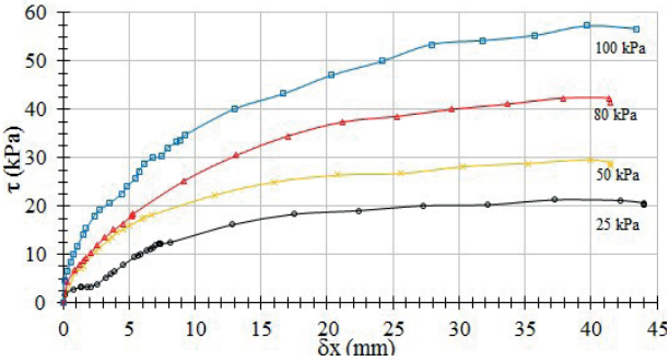
Figura 4: Deslocamento horizontal versus tensão cisalhante - M10%
