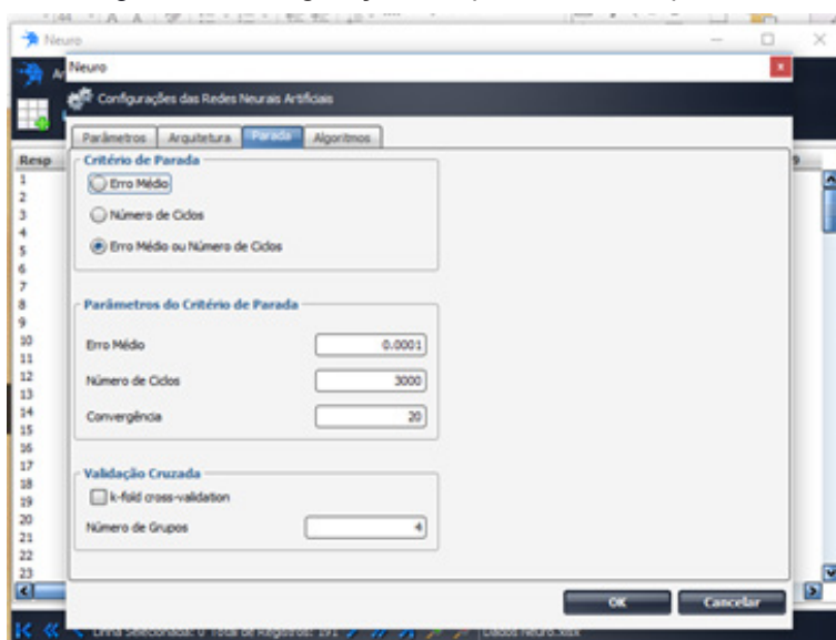
Figura 31: Configuração dos parâmetros de parada
