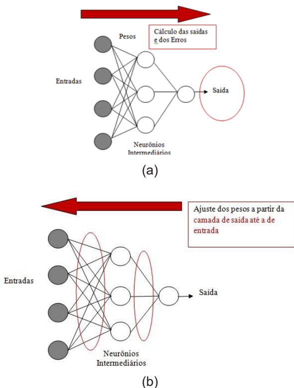
Figuras 20a e 20b: Fase forward do algoritmo backpropagation e Fase backward do algoritmo backpropagation.
