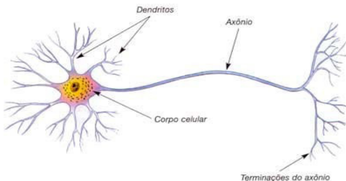
Figura 11: Modelo de um neurônio biológico
