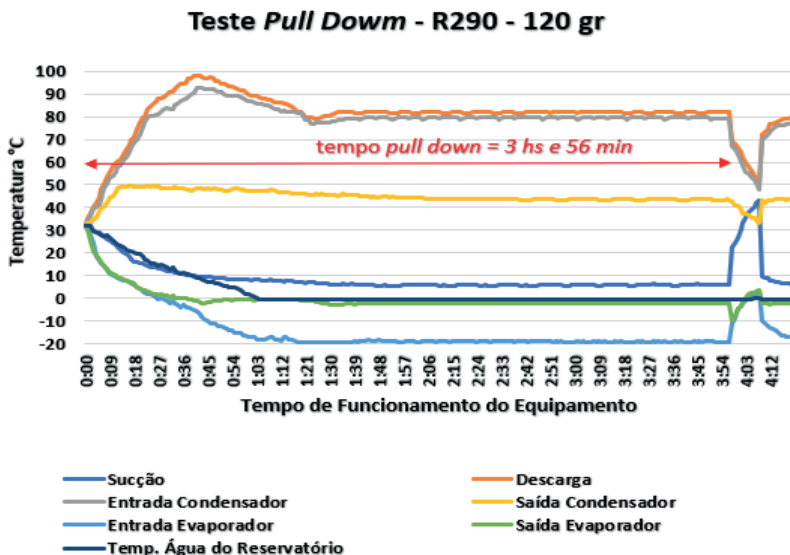
Figura 4 – Gráfico da variação de temperatura no equipamento com gás R290.
