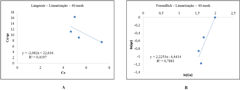
Figura 8. Isoterma de adsorção de Cr (VI) segundo o modelo de Langmuir para a farinha ativada de casca de laranja (FA) com granulometria de 40 mesh (A) e segundo o modelo de Freundlich para FA e 40 mesh (B). Fonte: Próprios autores.
