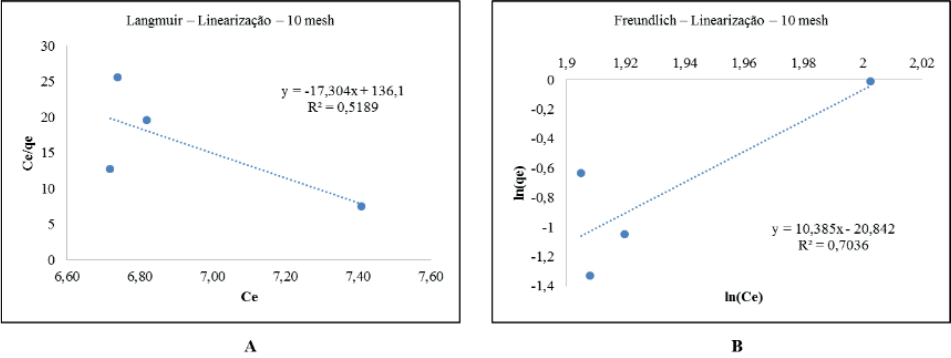
Figura 7. Isoterma de adsorção de Cr (VI) segundo o modelo de Langmuir para a farinha ativada de casca de laranja (FA) com granulometria de 10 mesh (A) e segundo o modelo de Freundlich para FA de 10 mesh (B). (Fonte: Próprios autores.)
