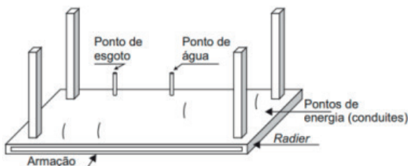
Figura 7 – Fundação Radier (Fonte: SALGADO, 2019)
