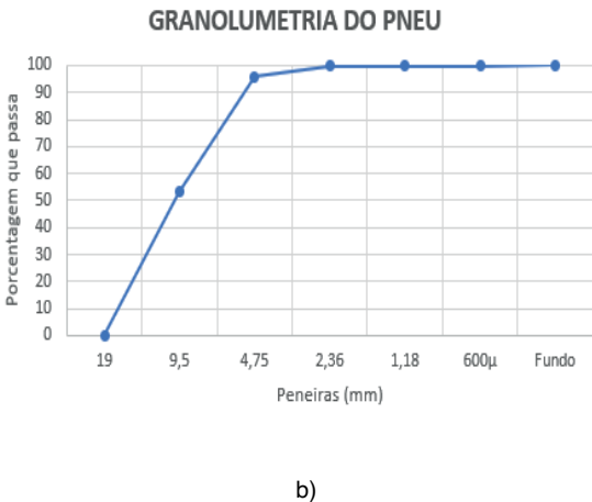
Figura 1 – Granulometria: a) Brita; b) Pneu. Fonte: Autores, 2022.
