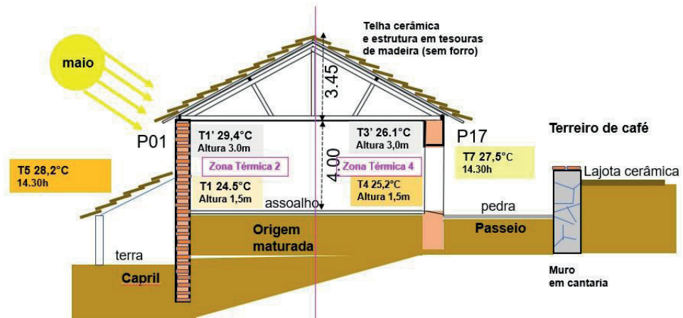
Figura 5. Corte esquemático do ambiente Origen Maturada onde foram coletadas as condições termo-higrométricas e as temperaturas termográficas. (Fonte: Próprio Autor, 2022).
