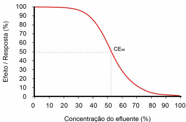
Figura 2. Representação gráfica hipotética da curva sigmóide dose-resposta. A concentração do efluente é determinada pela porcentagem ou outra unidade de medida de concentração do efluente. O valor de CE50 pode ser estimado por meio de interpolação do gráfico.
