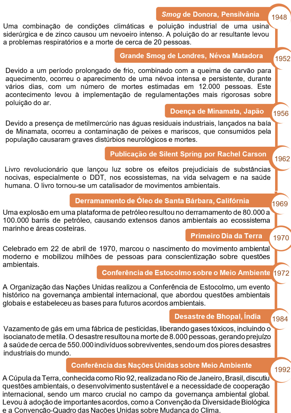
Figura 1. Linha do tempo com relato dos principais acontecimentos de tomada de consciência ambiental entre a Revolução Industrial e a Conferência das Nações Unidas.
