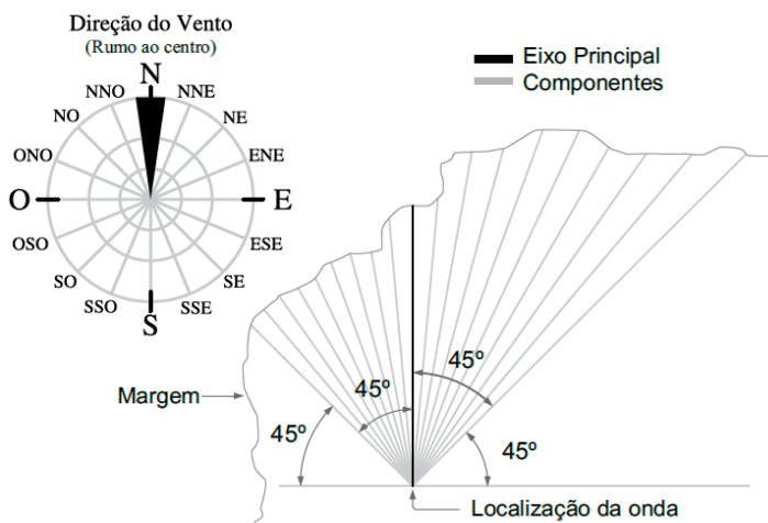
Figura 1: Traçado conceitual de fetch efetivo para a direção norte
