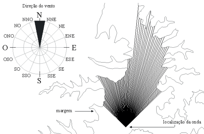
Figura 3 - fetch esquemático para a direção norte
