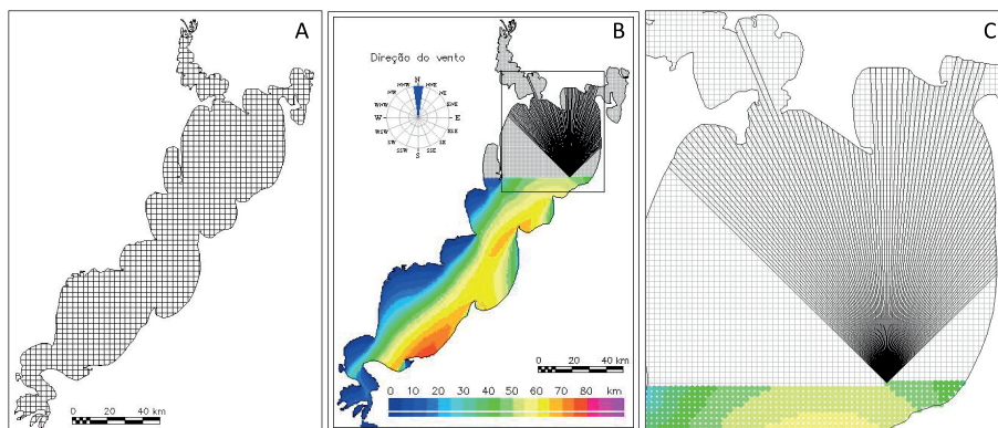
Figura 4 - (a) geração de uma malha estruturada quadrangular para a lagoa dos patos; (b) processamento propositalmente interrompido para mostrar os nós da malha sendo percorridos; (c) ampliação de parte da figura b
