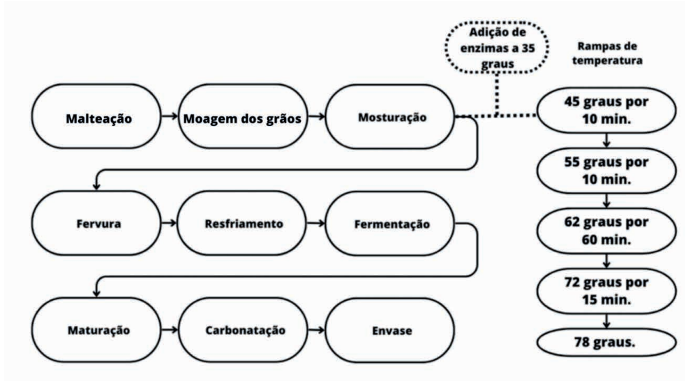
Figura 2. Fluxograma das etapas de processo cervejeiro
