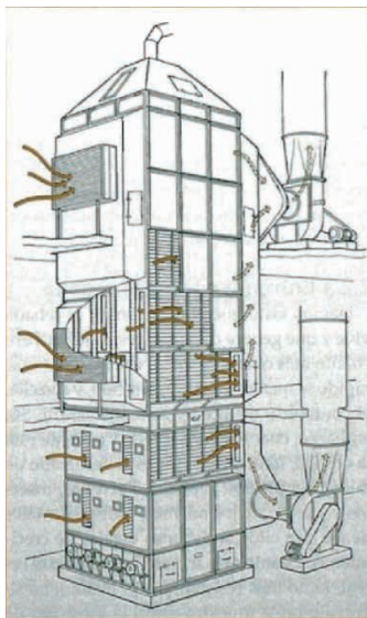
Figura 6. Estação de secagem da malteação. (KUNZE, W. 2019)
