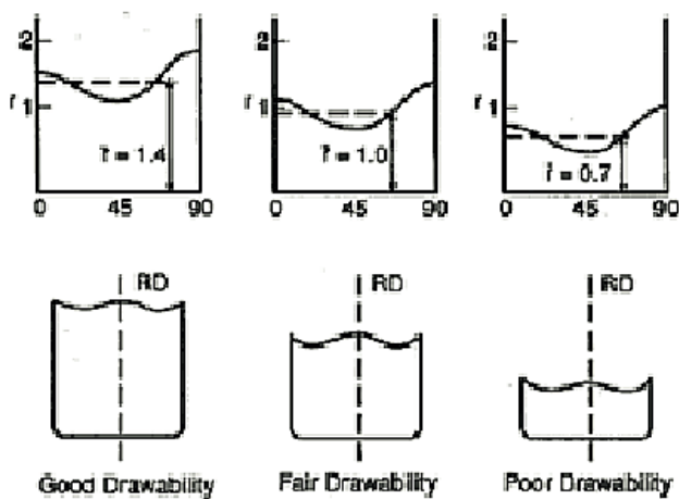
Figura 12: Anisotropia planar.
