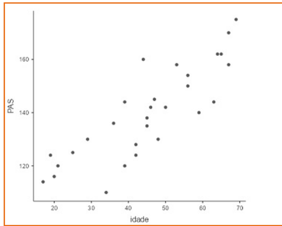
Figura 63. Diagrama de dispersão entre Pressão arterial sistólica
