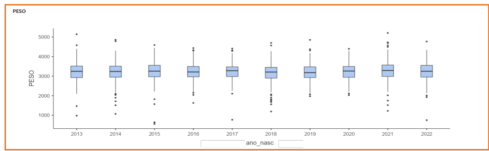
Figura E6.1.2. Boxplot da variável peso ao nascer segundo ano de nascimento
