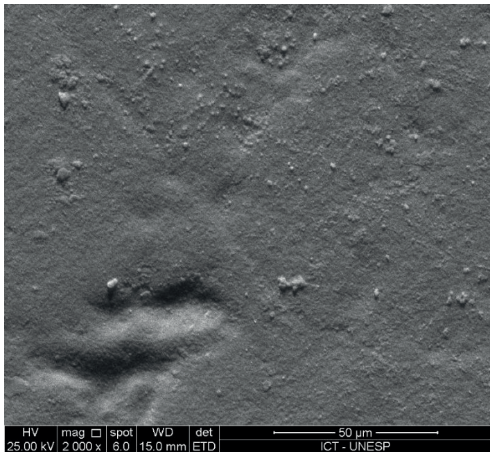
Figura 9 – Microscopia Eletrônica de Varredura da cerâmica Celtra Duo cristalizada por energia de micro-ondas com aumento de 2000x Fonte: Elaborado pelo autor.
