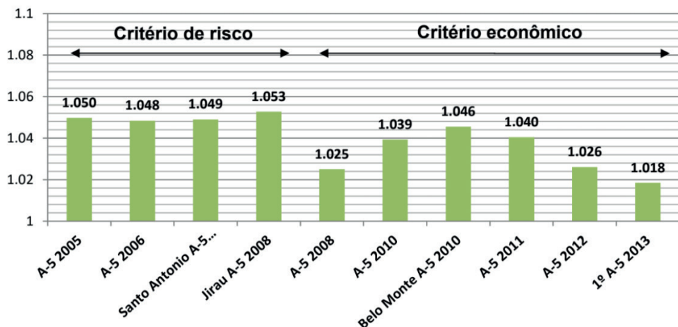
Figura 5.1 – Relação entre bloco hidráulico e energia firme para diversos leilões de energia. Elaborada pelo autor com base em [58;59;114 – 120].
