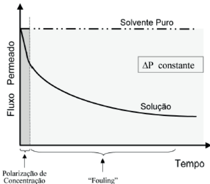
Figura 3.7. Variação esquemática do fluxo de permeado com o tempo de operação ocasionada por polarização de concentração e incrustação em operação tangencial (Habert, 2006).
