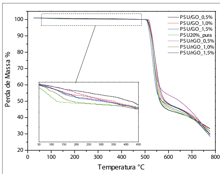
Figura 5.7. Termograma (TGA) das membranas compósitas sintetizadas
