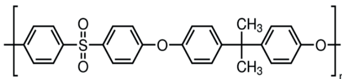
Figura 3.11. Fórmula estrutural da unidade de repetição da polisulfona (Udel, 2015).
