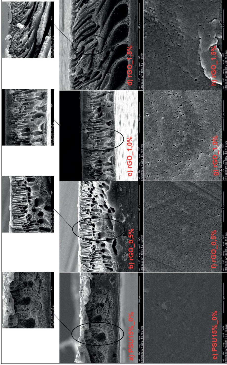
Figura 5.3. Fotomicrografia da superfície (e,f,g,h; magnificação:100.000x) e seção transversal (a,b,c,d; magnificação:1.500x) das membranas de óxido de grafeno reduzido.
