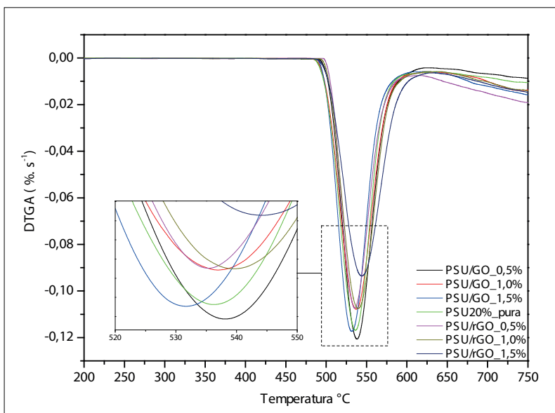
Figura 5.8. Termogramas (DTGA) das membranas compósitas
