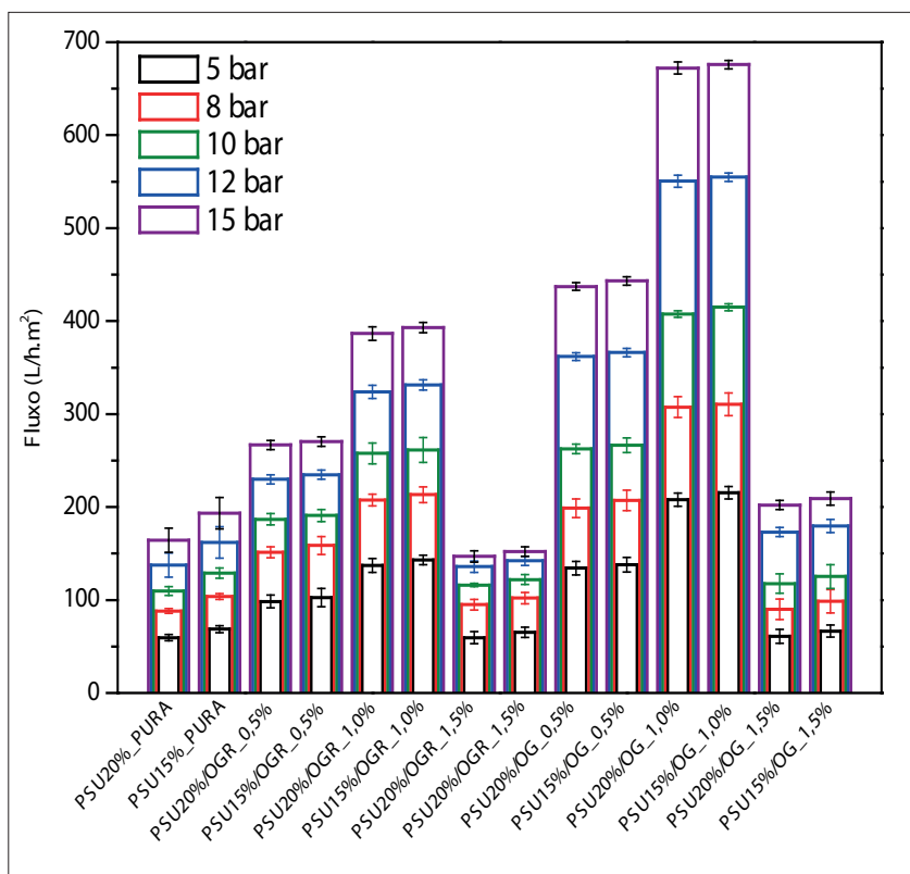
Figura 5.14. Fluxo de permeado a água em diferentes pressões ( 5 \text{ bar} \leq P \leq 15 \text{ bar} ; T=25 \pm 2^\circ\text{C} ) para as membranas compósitas estudadas (Barra de erro: desvio padrão, n= 3 ).
