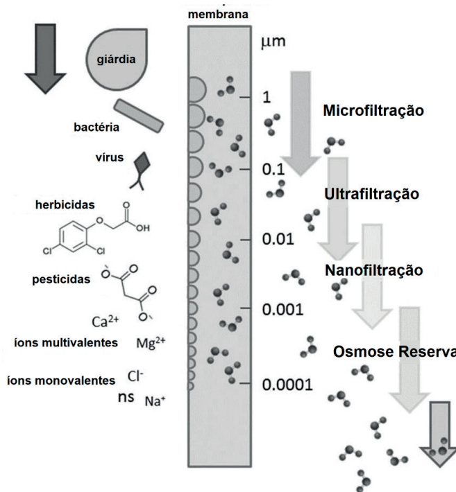
Figura 3.2. Tipos de membranas, variação de tamanho de poros e contaminantes de água removidos por cada faixa de tamanho de poro (Adaptado de Rodriguez-Narvaez et al., 2017).
