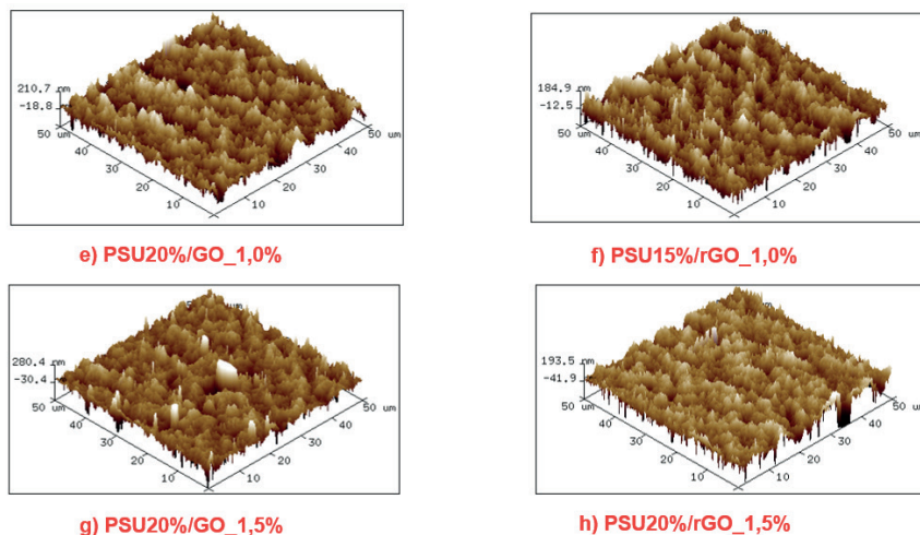
Figura 5.4. Morfologia de superfície tridimensional, AFM das membranas preparadas em a) PSU20%, b) PSU15%, c) GO_0,5%, d) rGO_0,5%, e) GO_1,0%, f) rGO_1,0%, g) GO_1,5%, h) rGO_1,5%.
