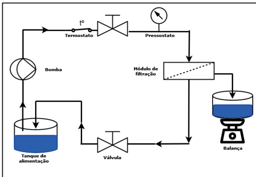
Figura 4.5. Esquema de filtração por ultrafiltração de fluxo tangencial
