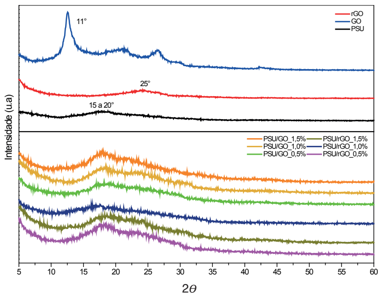
Figura 5.6. Difratogramas de DRX para PSU sem carga e com carga de GO e rGO e membranas compósitas.
