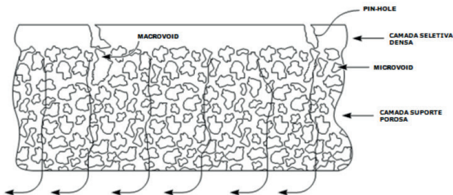
Figura 3.10. Membrana com defeitos (Baker, 2004).
