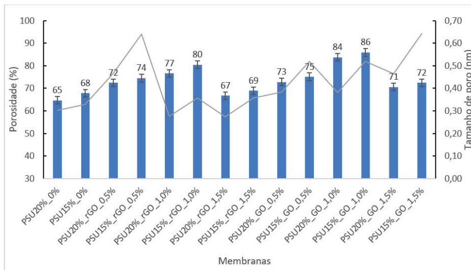
Figura 5.13. Porosidade das diferentes membranas compósitas produzidas. (Barra de erro: desvio padrão, n= 5).
