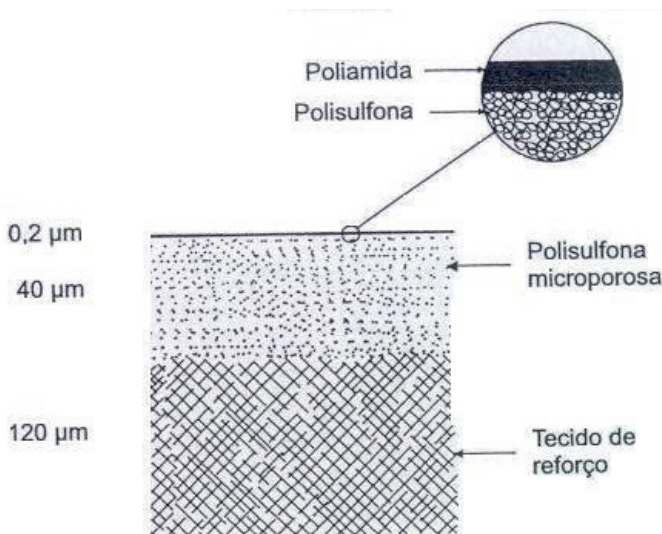
Figura 3.3. Estrutura de membrana polimérica (Schneider; Tsutiya, 2001).
