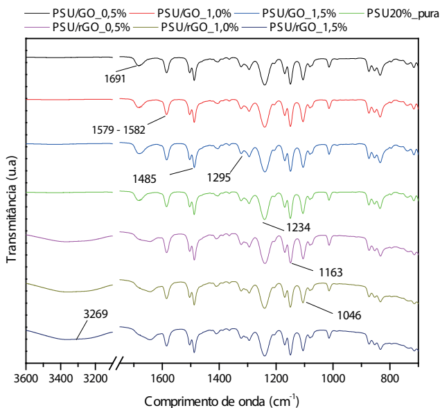
Figura 5.5. Espectroscopia de infravermelho das membranas PSU/GO e PSU/rGO.
