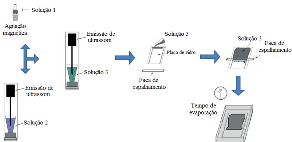
Figura 4.3. Representação esquemática do preparo de solução, espalhamento e imersão da solução de fundição. Adaptado de Ohland (2015).
