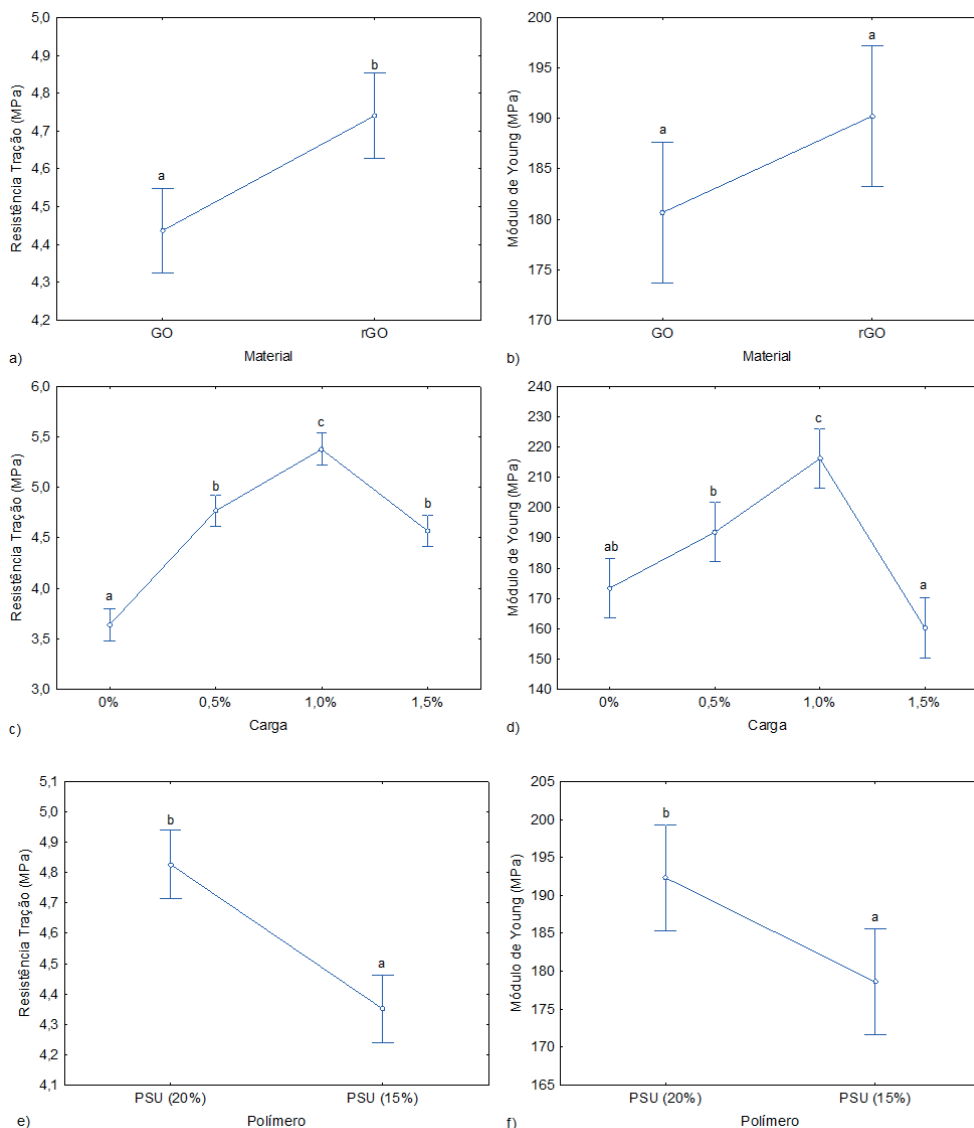
Figura 10.1 –Efeitos isolados nas propriedades mecânicas, resistência a tração (a); (c); (e); módulo de Young (b);(d); (f).
