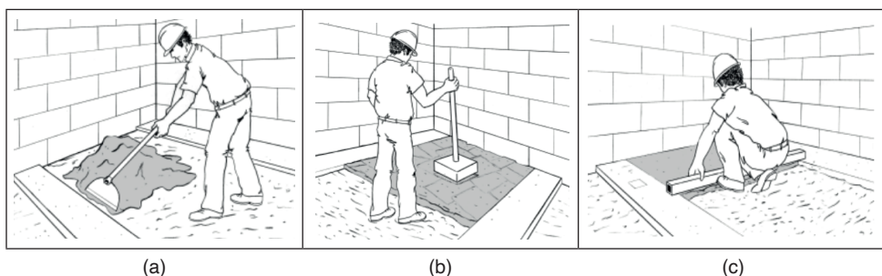
Figura 53: Espalhamento de argamassa (a), compactação (b) e sarrafeamento entre as mestras (c)
