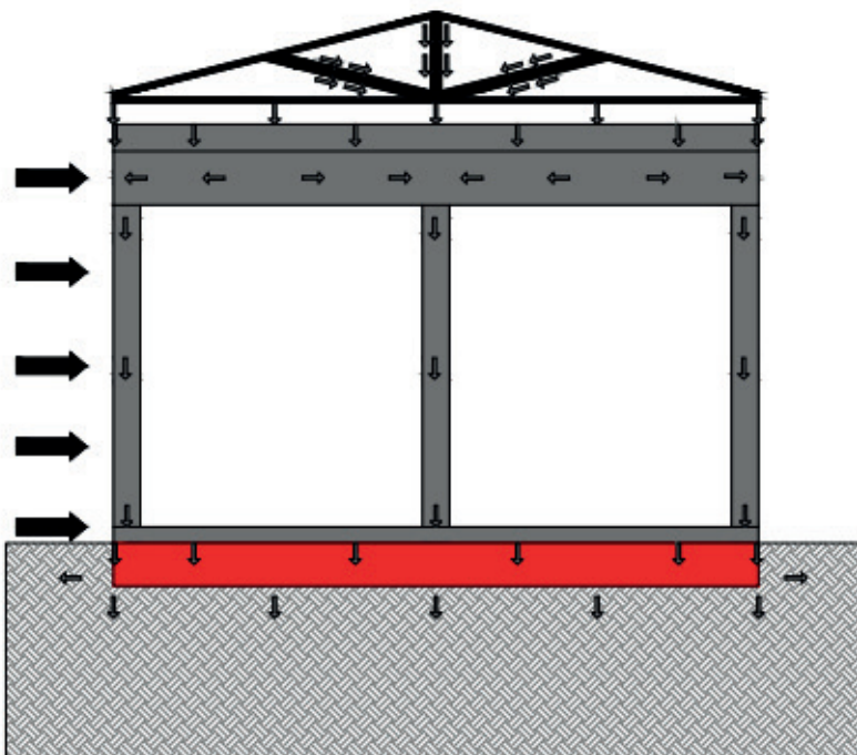
Figura 17 - Fundação tipo radier
