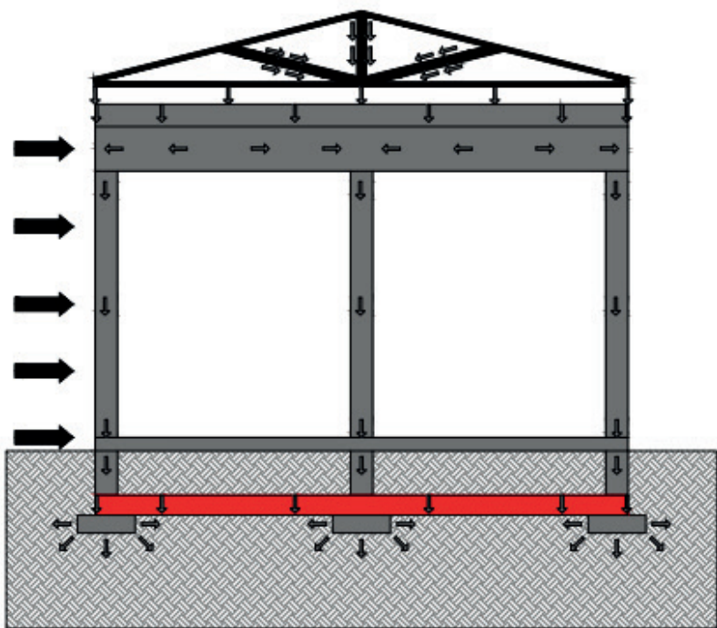
Figura 16 - Fundação tipo sapata isolada
