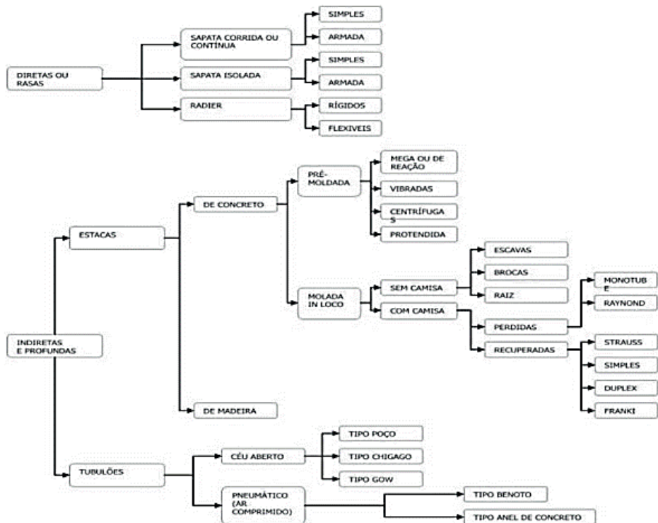
Figura 14 - Tipos de fundação
