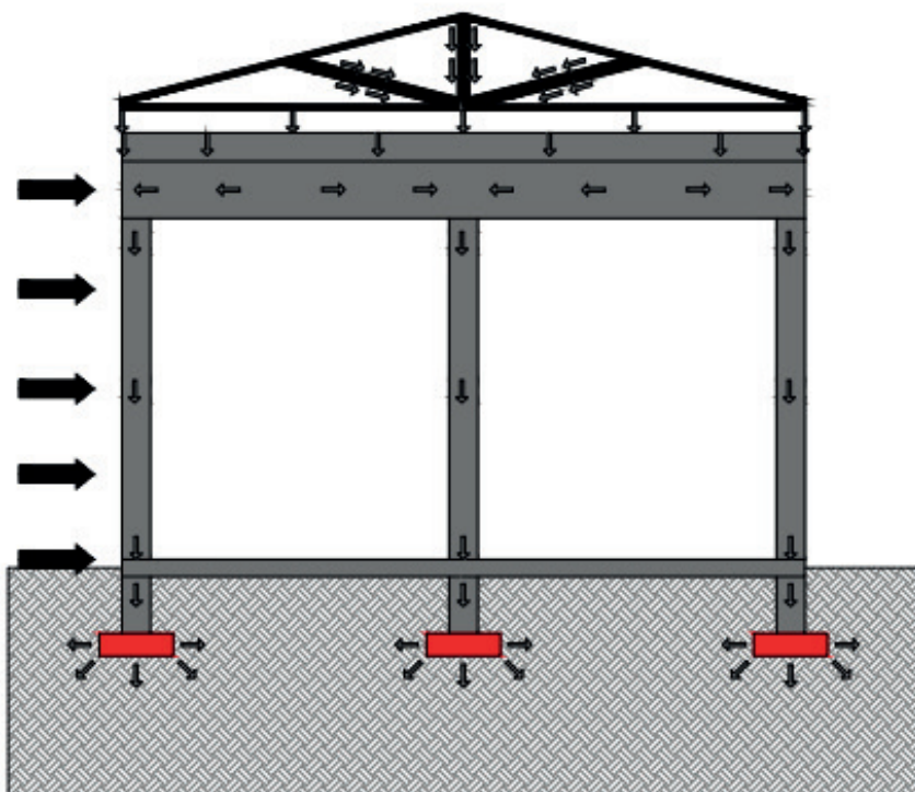
Figura 15 - Fundação tipo sapata isolada
