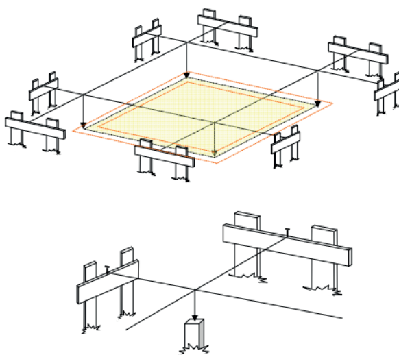
Figura 13 - Locação por cavaletes
