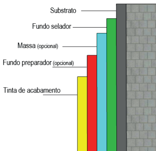
Figura 54: Principais constituintes do sistema de pintura
