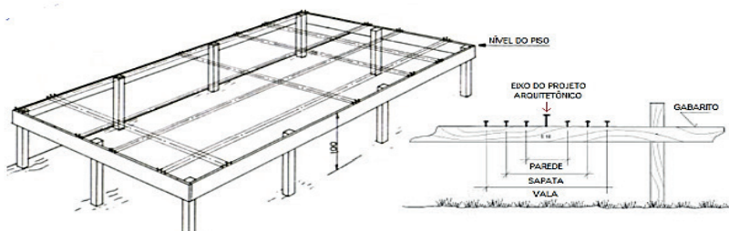
Figura 11 - Detalhamento de locação por gabarito
