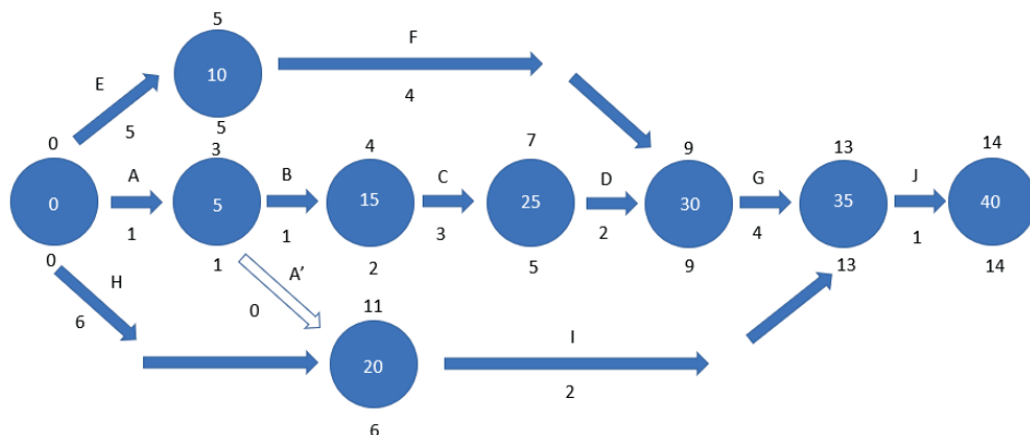
Figura 81 - Tempo Mais Tarde
