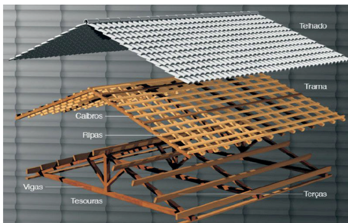
Figura 40 - Sistema estrutural de cobertura
