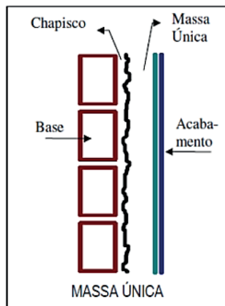
Figura 52 - Camadas de revestimento de argamassa de vedação em massa única.
