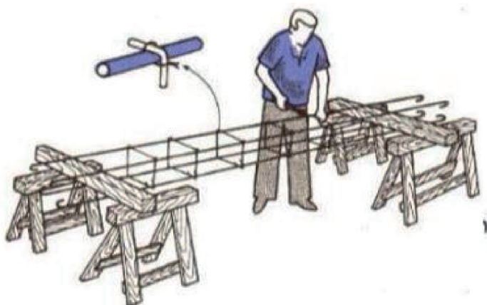
Figura 30 - Procedimento de armação das barras de ferro
