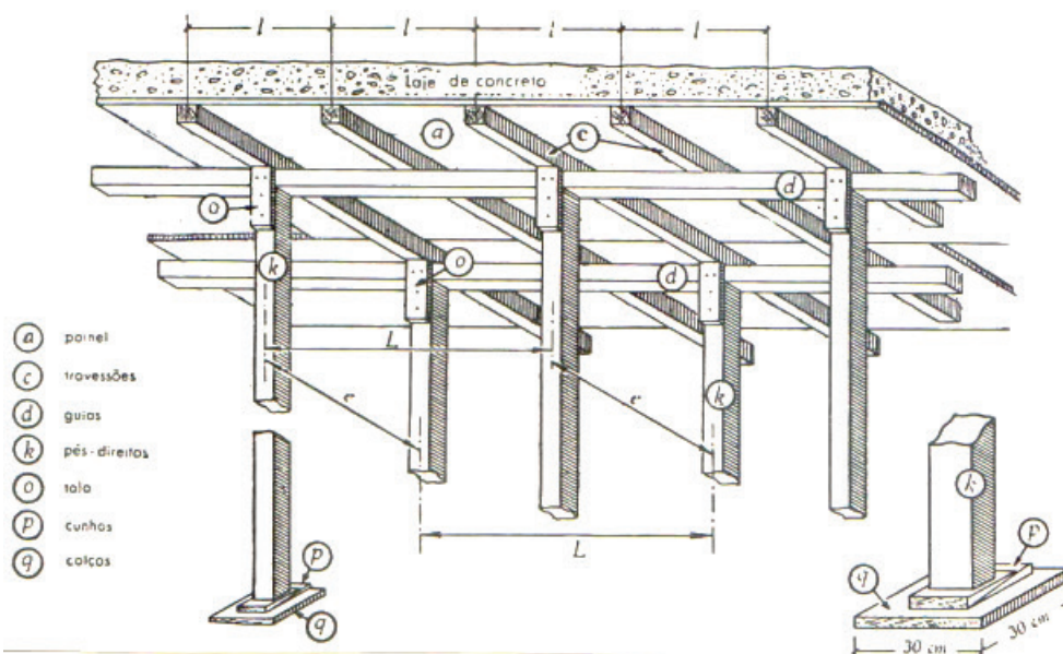
Figura 24 - Esquema de fôrma convencional para laje, utilizando-se travessões e guias
