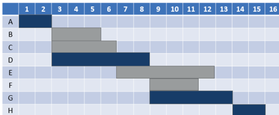
Figura 65 - Cronograma de obras em gráfico de barras (caminho crítico)
