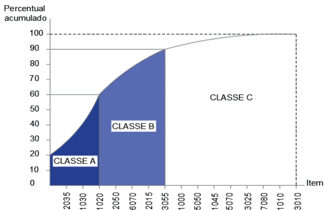
Figura 85 - Criticidade dos Itens de Estoque
