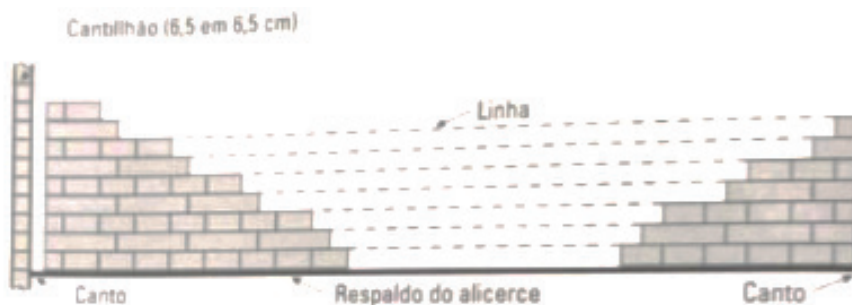
Figura 35 - Sistema de orientação para alvenaria
