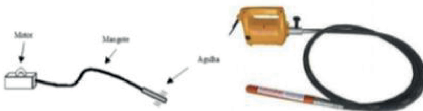
Figura 33 - Aparelho que realiza o processo de vibração para homogeneizar a concretagem
