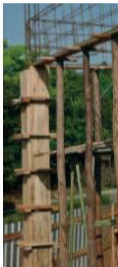
Figura 20 - Fôrma de madeira para pilares
