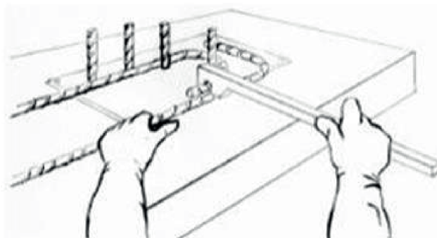
Figura 28 - Procedimento de dobragem das barras de ferro
