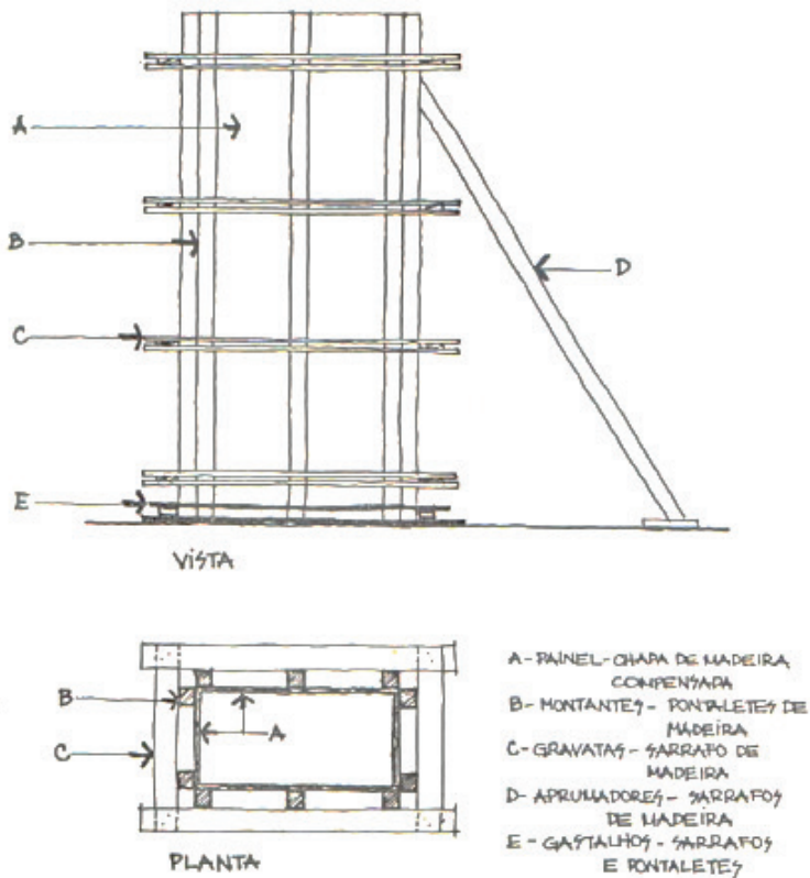
Figura 21 - Esquema de fôrma convencional para pilar
