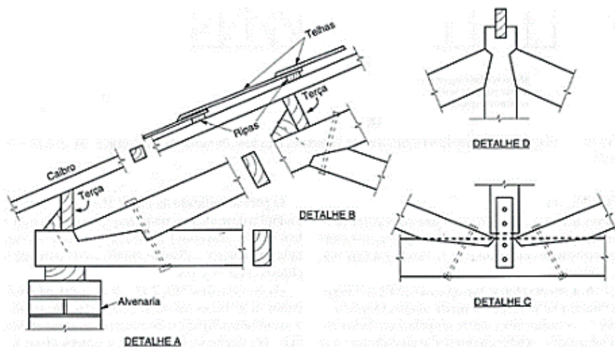
Figura 45 - Ligação de entalhe
