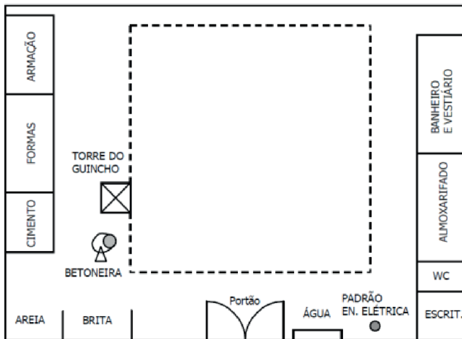
Figura 10 - Layout de canteiro de obras
