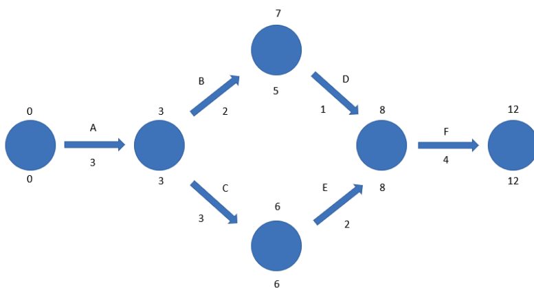
Figura 59 - Diagrama de rede
