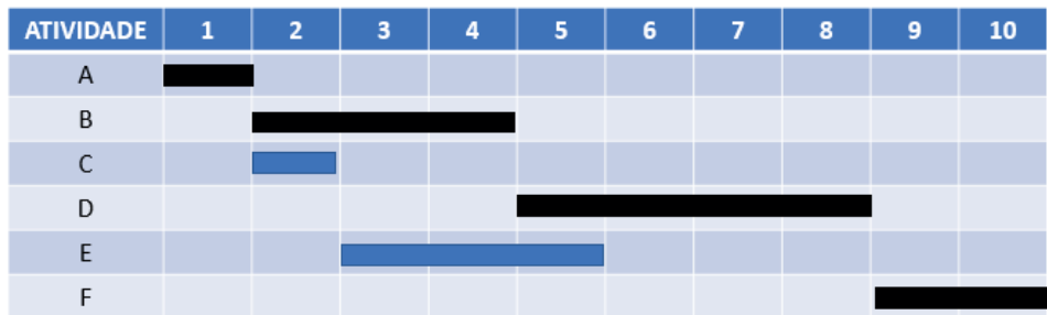
Figura 77 - Caminho crítico no cronograma
