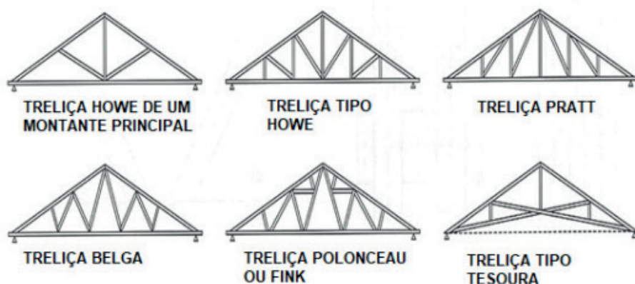
Figura 41 - Sistemas de treliças triangulares
