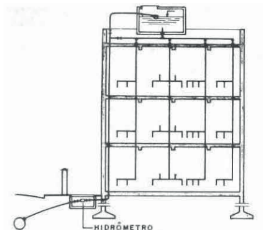
Figura 46 - Representação de sistema abastecimento indireto, sem bombeamento
