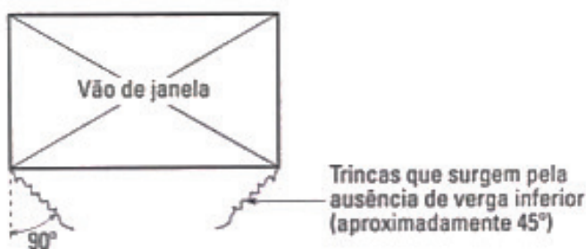
Figura 39 - Demonstração dos esforços sem a presença das vergas em vãos
