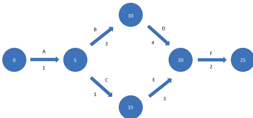
Figura 75 - Rede com atividades e durações: diagrama de flechas
