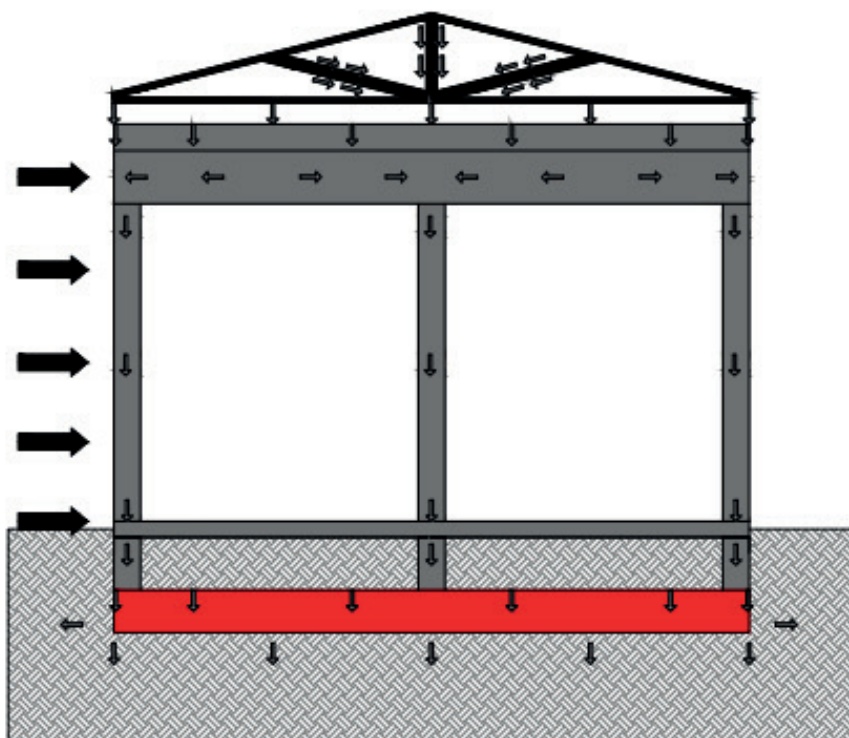
Figura 18 - Fundação tipo sapata corrida
