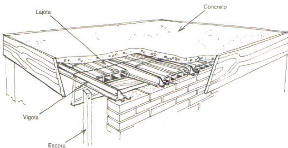
Figura 26 - Esquema de laje mista usualmente empregada em edifícios de múltiplos pavimentos
