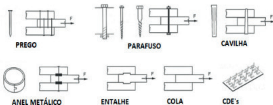
Figura 44 - Exemplos de ligações em peças de madeira
