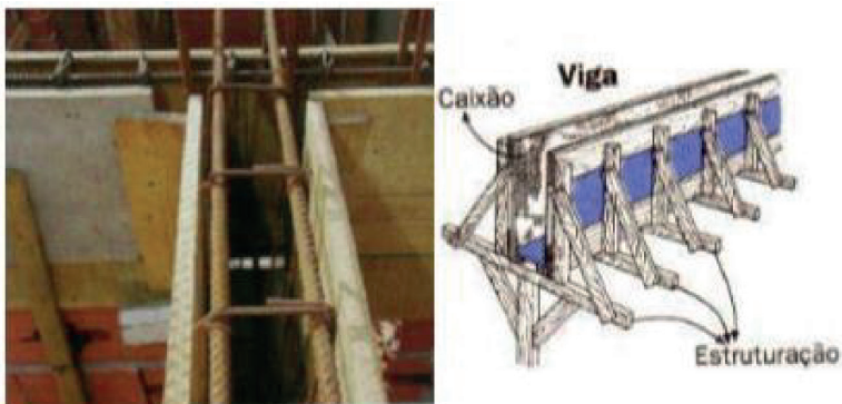
Figura 22 - Fôrma de madeira para vigas
