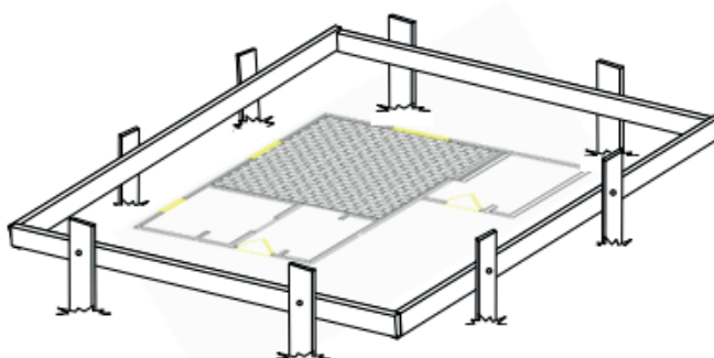
Figura 12 - Locação por gabarito
