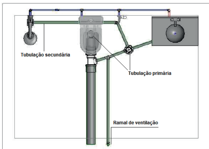
Figura 48 - Tubulação primária e secundária
