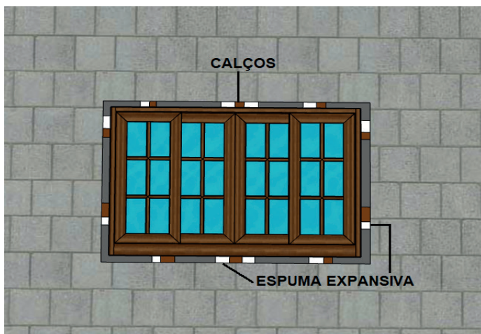
Figura 49 - Pontos de aplicação de espuma expansiva em janelas
