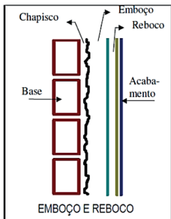
Figura 51 - Camadas de revestimento de argamassa de vedação com emboço e reboco
