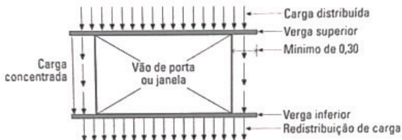
Figura 38 - Demonstração dos esforços com a presença das vergas em vãos
