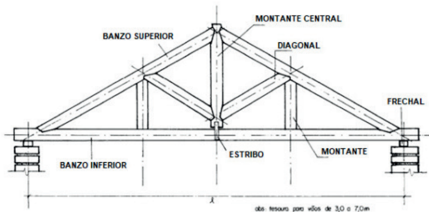
Figura 42 - Sistema de tesoura tipo Howe
