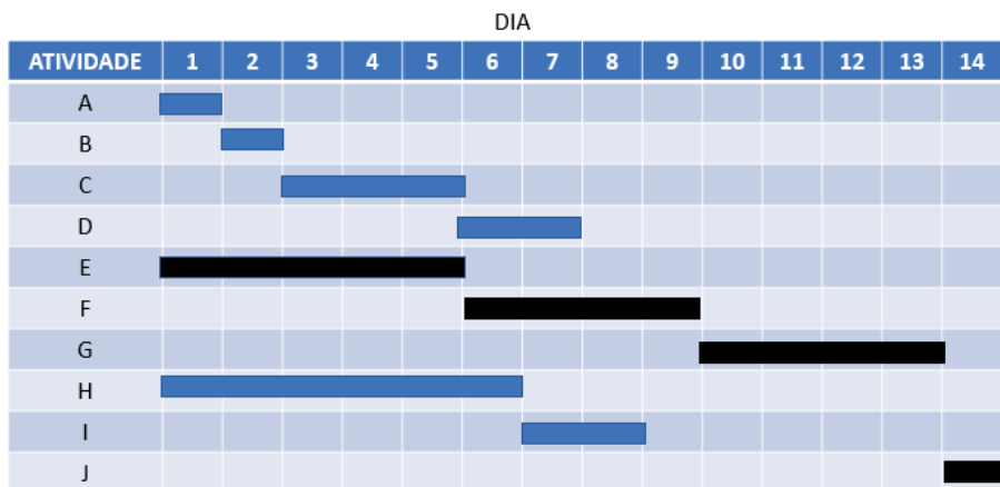
Figura 83 - Cronograma Mais Cedo Fonte: Próprio autor (2020).
