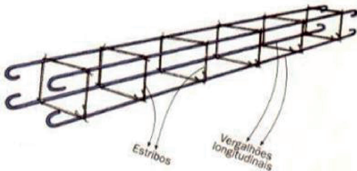
Figura 31 - Armadura finalizada e pronta para ser posicionada
