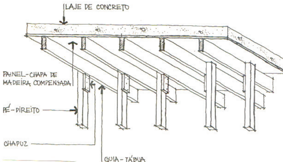
Figura 25 - Esquema de fôrma convencional para laje, utilizando-se apenas guias
