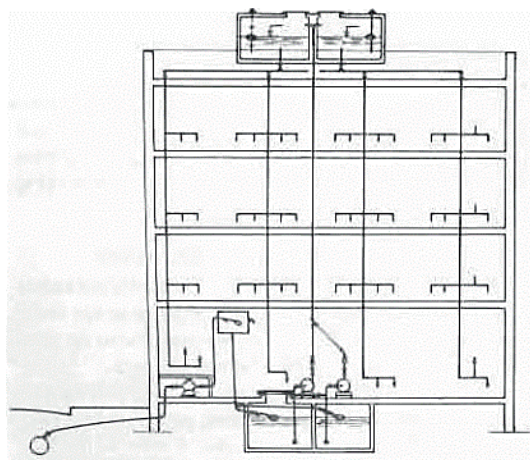
Figura 47 - Representação de sistema de abastecimento indireto, com bombeamento
