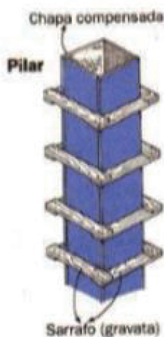
Figura 20 - Fôrma de madeira para pilares
