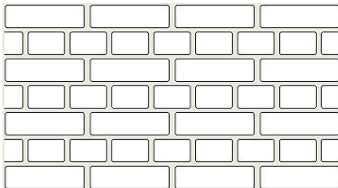
Figura 37 - Amarração francesa de tijolos
