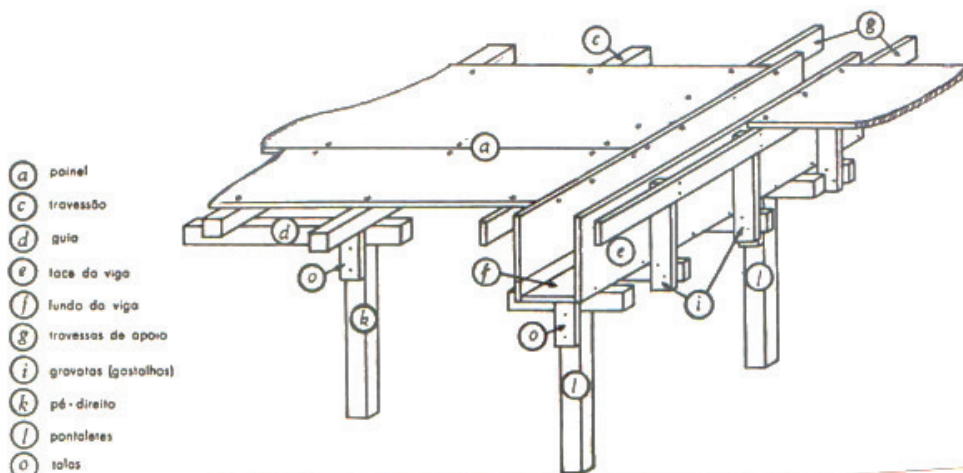
Figura 23 - Esquema de fôrma convencional para viga
