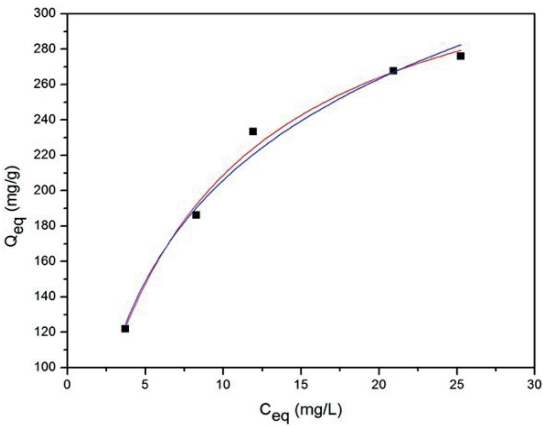
Figura 8. Dados experimentais de equilíbrio de adsorção do Metamizol (símbolos vazados) e ajustes dos modelos de — Langmuir e — Temkin. Concentração de carvão ativado: 0,5 g/L; t = 240 min; T = 20\text{ }^{\circ}\text{C} \pm 1 .
