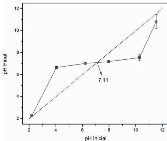
Figura 3. Curva de pH de ponto de carga zero (pHPCZ) do carvão ativado em pó.
