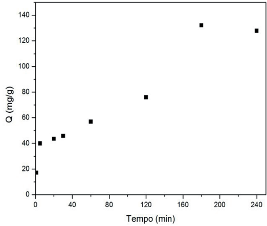
Figura 6. Cinética de adsorção do Metamizol com carvão ativado: C_{\text{inicial}} = 100 \text{ mg/L} ; C_{\text{carvão}} = 0,5 \text{ g/L} ; T = 20 \text{ }^{\circ}\text{C} ; \text{pH} = 6,40 .
