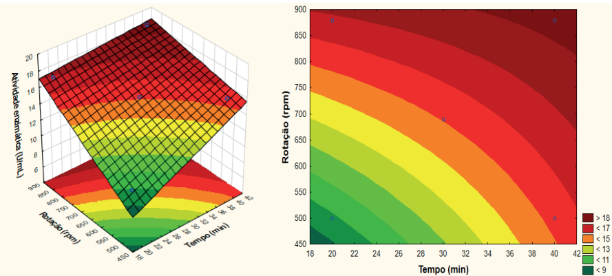
Figura 2 – Curvas de contorno da atividade enzimática vs velocidade; tempo via centrifugação.
