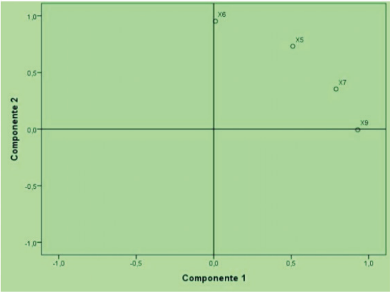
Figura 12: Gráfico de componentes en espacio rotado
