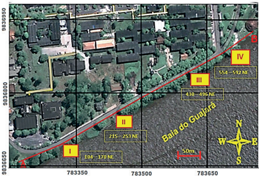
Figura 3. Centros dos quatro levantamentos de Eletrorresistividade
