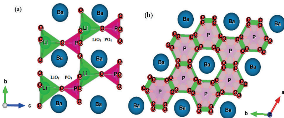
Figura 1: Estrutura do LiBaPO 4 na fase hexagonal com grupo P6 3 ao longo do eixo a (a) e ao longo do eixo c (b) ilustrando o ordenamento dos grupos tetraedros de LiO 4 e PO 4 entre os sítios de Ba.
