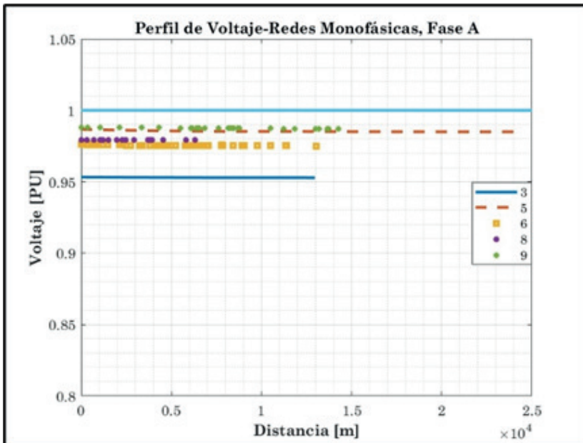
Figura 46. Perfil de voltaje, redes monofásicas conectadas a la fase A.
