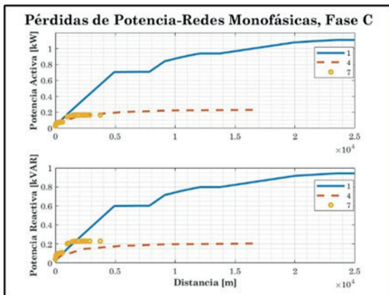
Figura 19. Pérdidas de potencia, redes monofásicas conectadas a la fase C.
