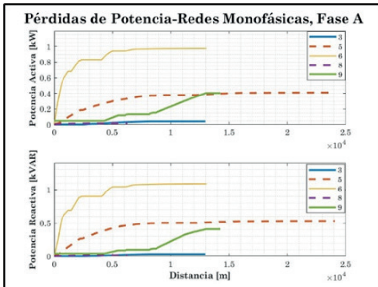
Figura 31. Pérdidas de potencia, redes monofásicas conectadas a la fase A.
