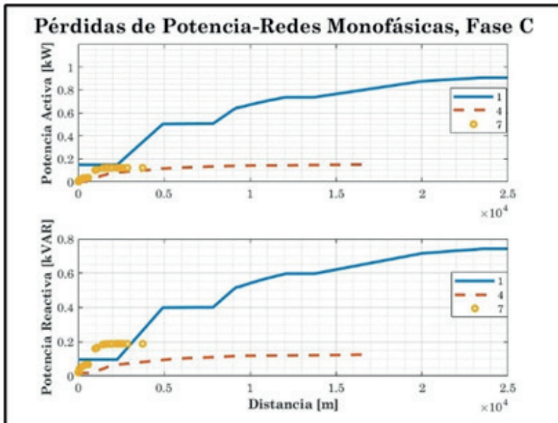
Figura 35. Pérdidas de potencia, redes monofásicas conectadas a la fase C.
