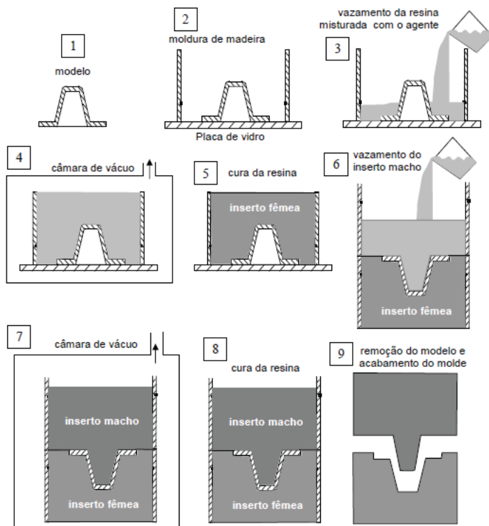
Figura 4 - Etapas de fabricação indireta de insertos para moldes de injeção.
