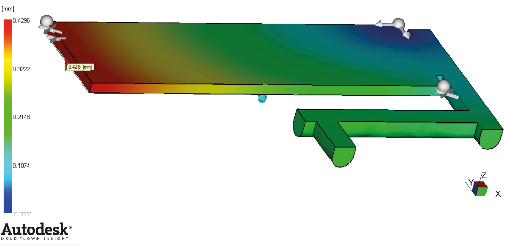
Figura 52 - Resultado do empenamento simulado para o PLA em molde VRE a 38°C para espessura de 3 mm.
