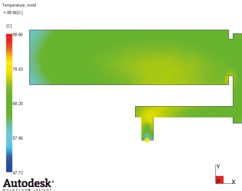
Figura 44- Resultado da temperatura nas paredes da cavidade na simulação da PA66 em molde VRE, após a extração.
