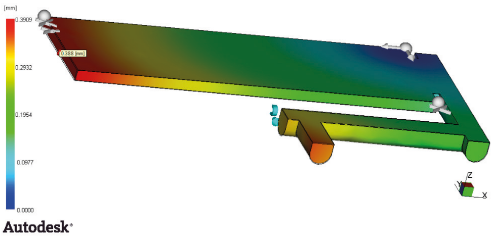
Figura 51 - Resultado do empenamento simulado para o PLA em molde VRE a 25°C para espessura de 3 mm.
