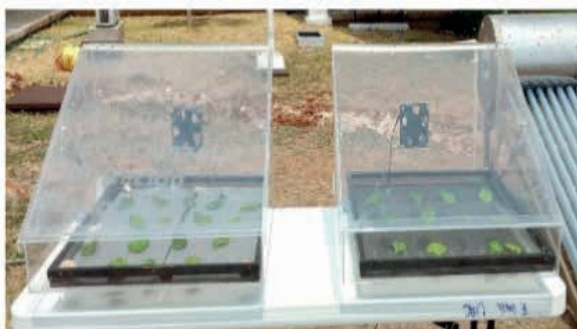
Imagen 1 Secador solar tipo gabinete
