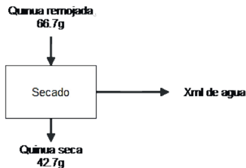
Figura 3. Balance de materia secado
