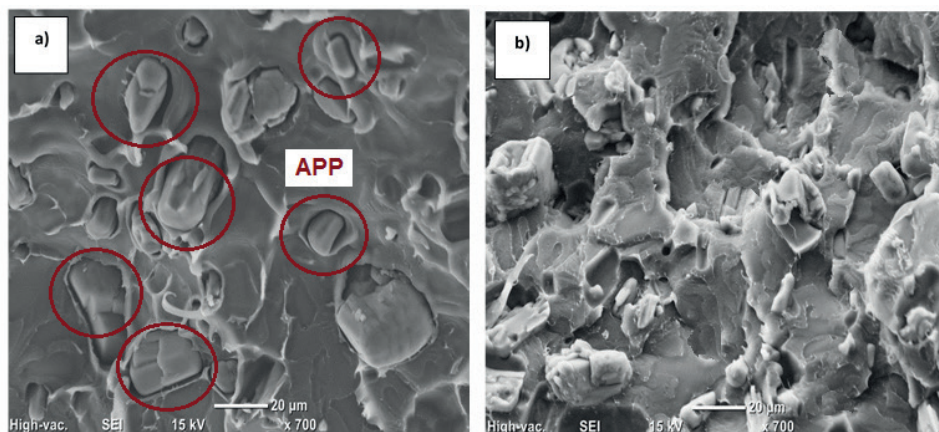
Figura 9. Imágenes SEM de la fractura por impacto de PLA/APP (15%) (a) PLA/PLA-g-APP (b).
