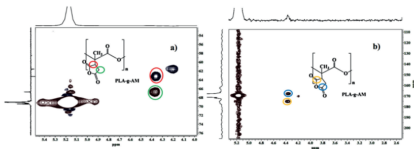
Figura 5. Espectros de RMN de correlación C-H (400 MHz) (a) HSQC y (b) HMBC de PLA-g-MA.
