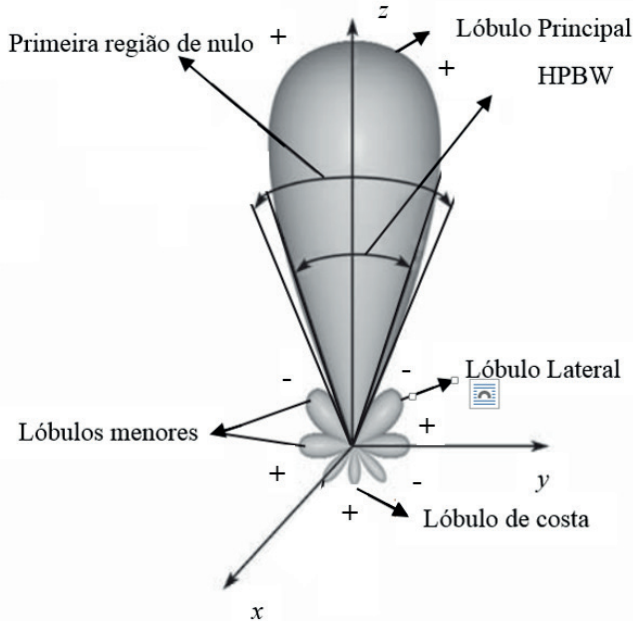
Figura 3. Exemplo do diagrama de irradiação [8].
