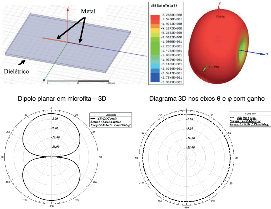
Figura 4. Dipolo planar com diagrama de irradiação 3D e 2D.
