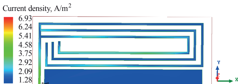
Figura 8. Desnsidade de corrente ( A/m^2 ) da antena PCB espiral flexível simulada.
