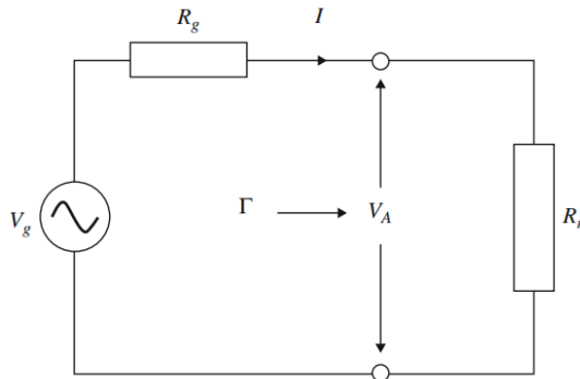
Figura 5. Circuito equivalente das perdas de uma antena com um gerador [26].
