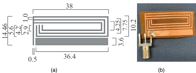
Figura 1. Antena PCB espiral flexível na forma da letra P: a) Simulada com as cotas em mm; b) Protótipo.
