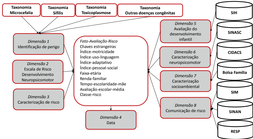
Figura 4. Esquema estrela multidimensional.
