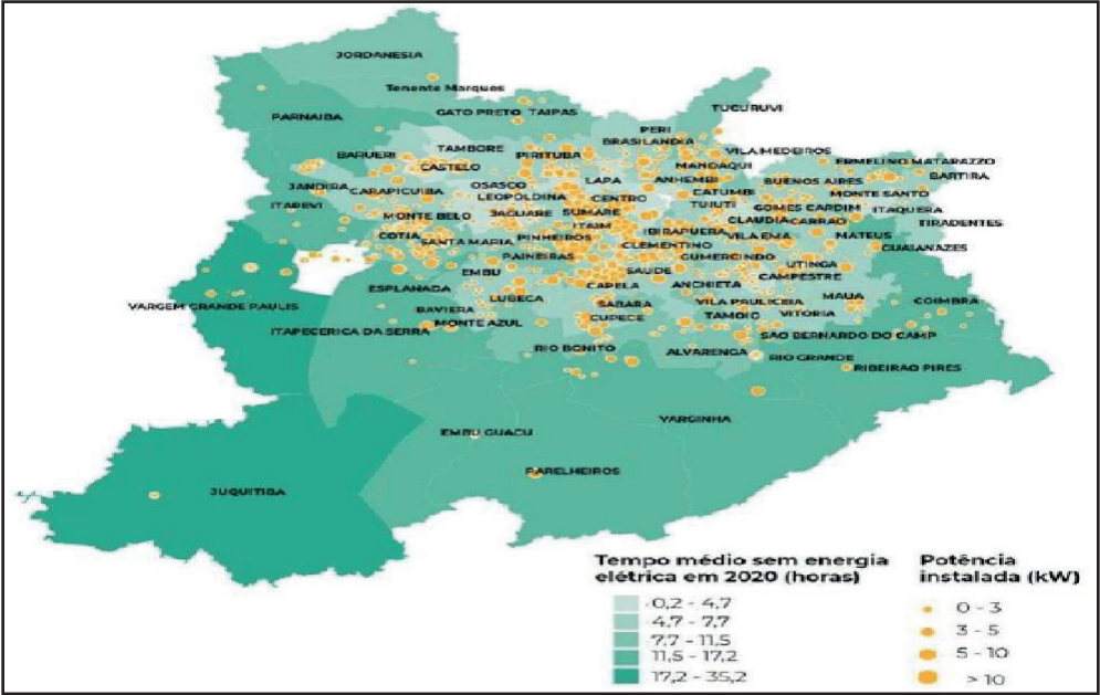
Figura 3. Localização das ligações de GD e tempo médio sem energia na área da Enel SP.
