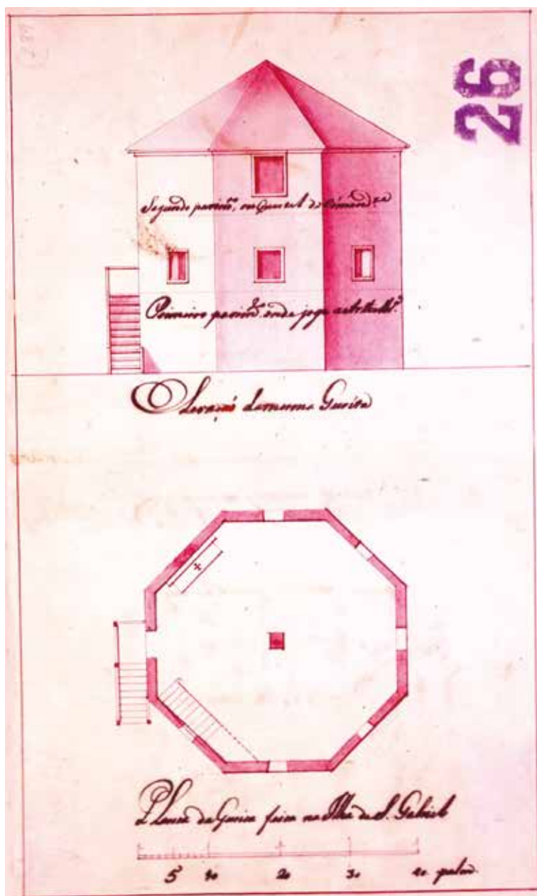
Figura 29 Planta da guarita localizada em uma ilha de São Gabriel com quartel do comandante no segundo pavimento e da artilharia no primeiro.
