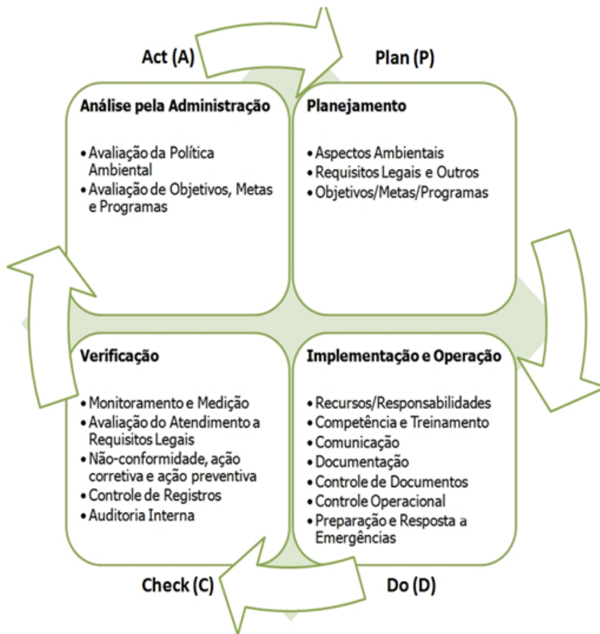
Figura 4 - Ciclo PDCA
